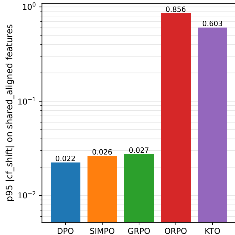
SmolLM3-3B
