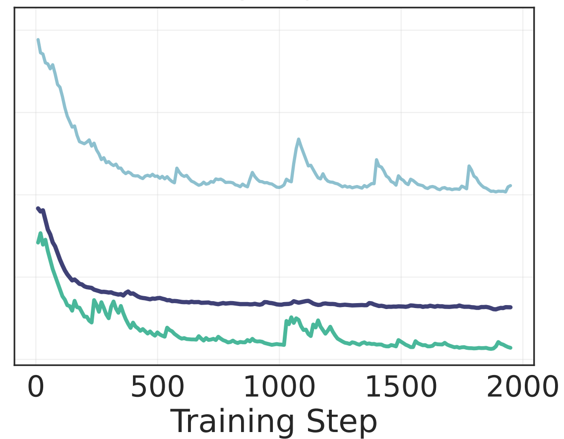
GRPO
