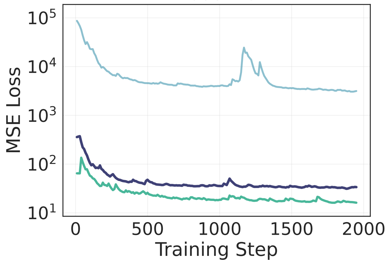
Baseline
