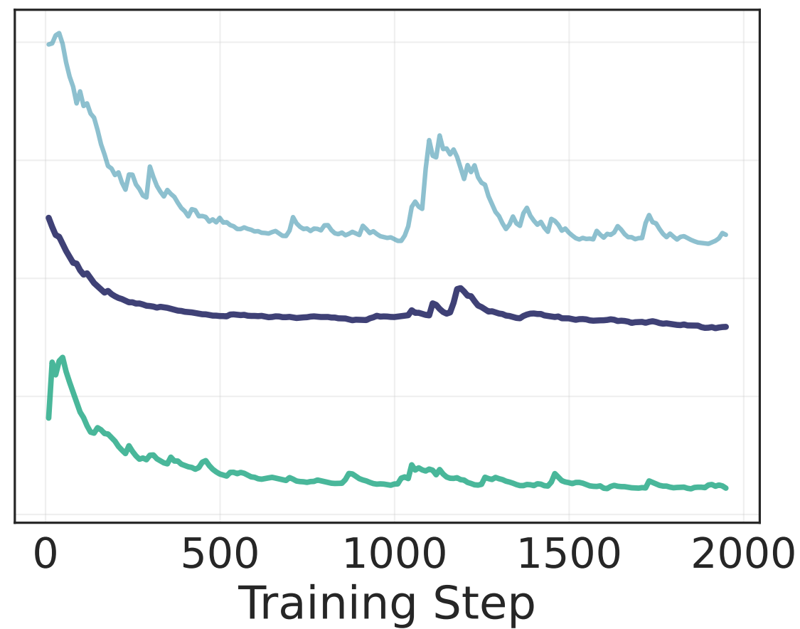
ORPO
