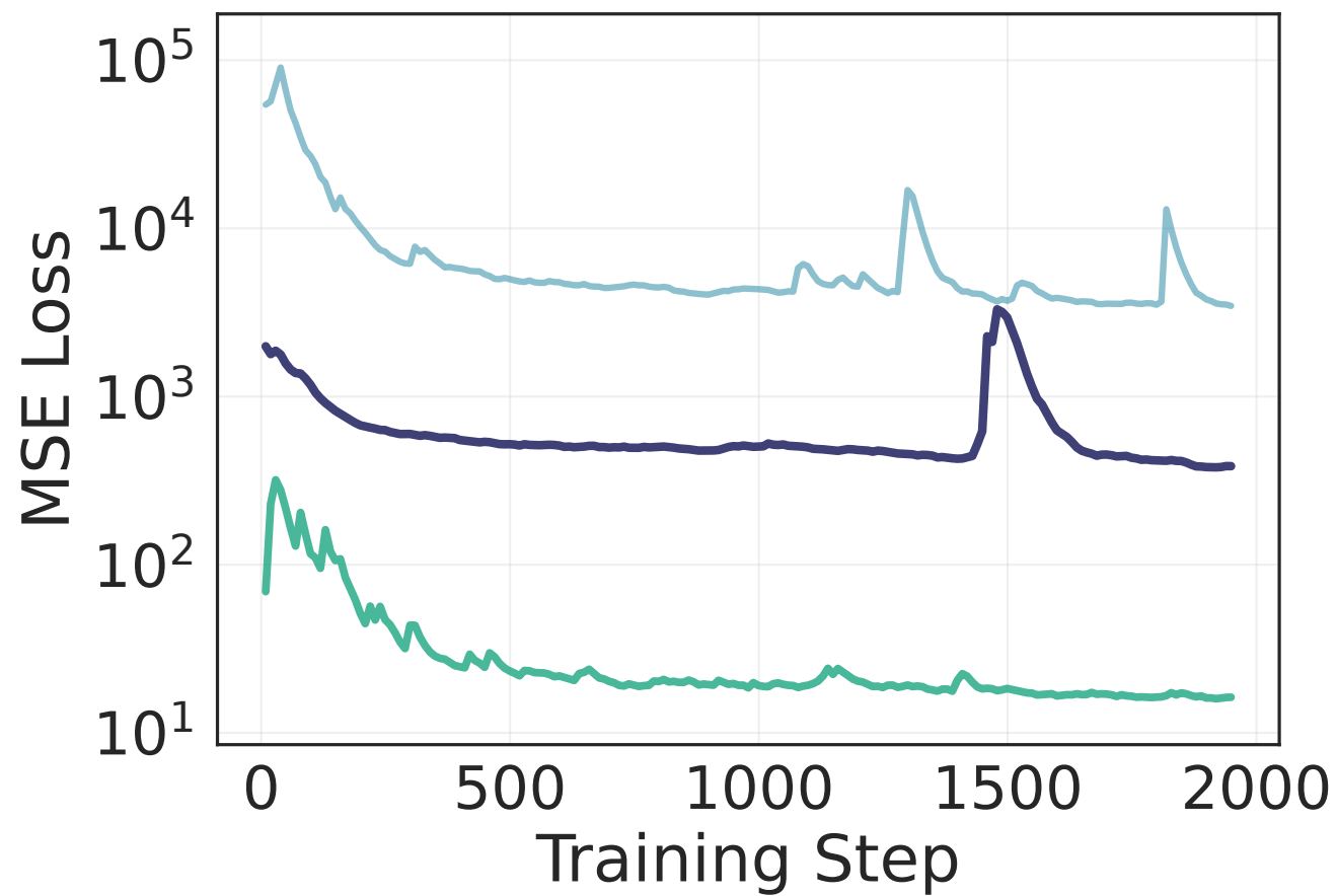
KTO
