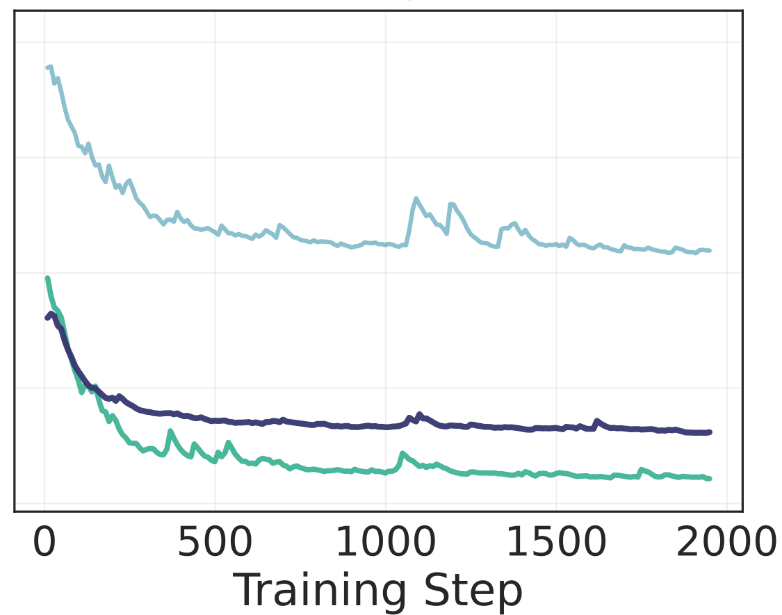
DPO
