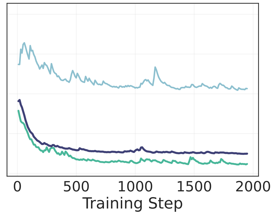
SimPO
