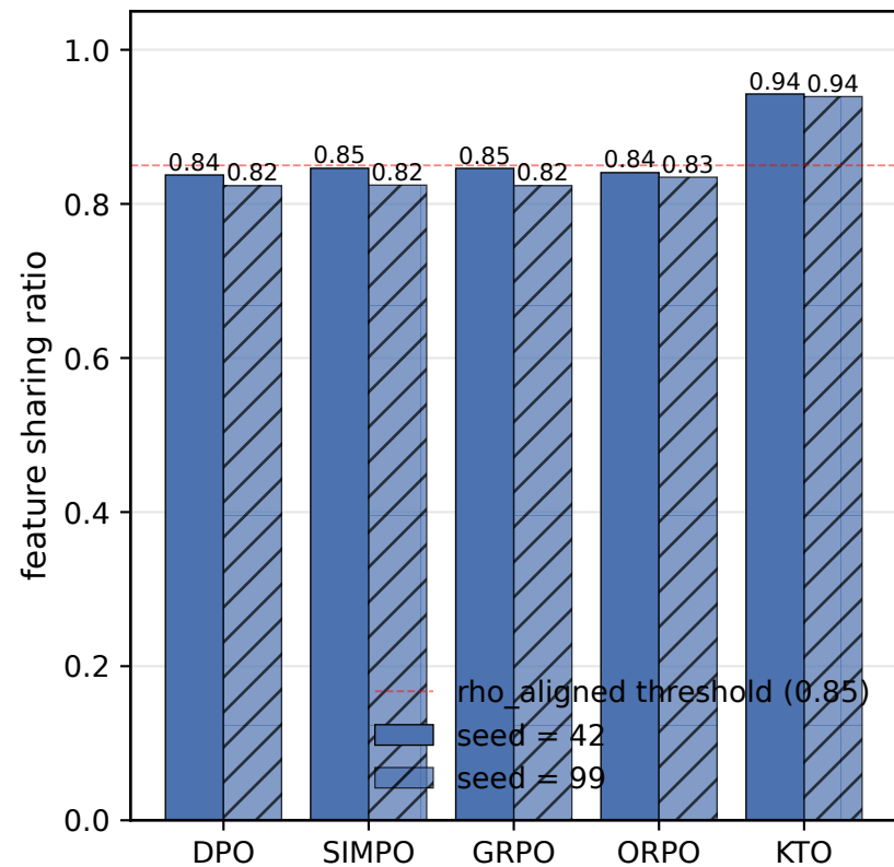
SmolLM3-3B
