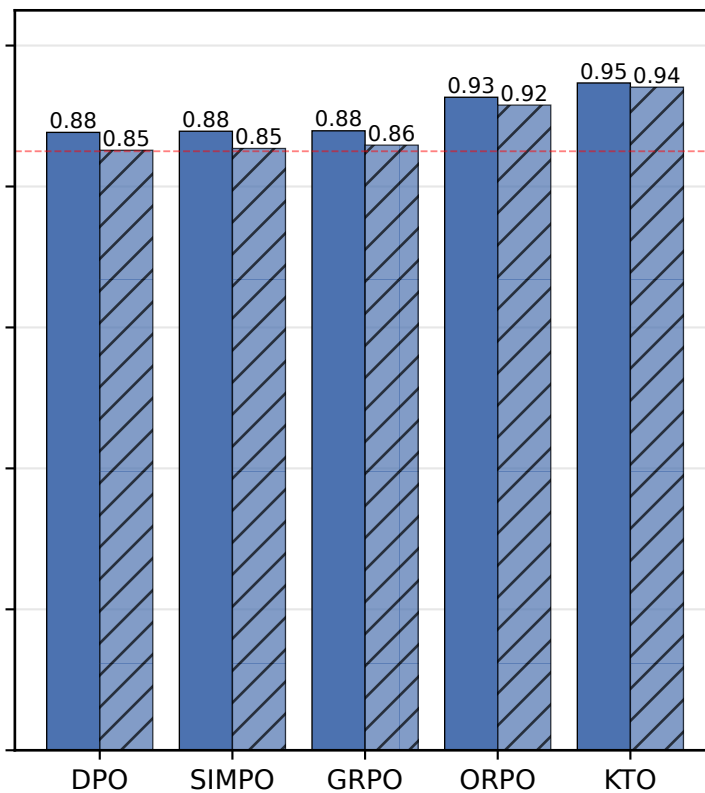
Llama-3.2-3B-Instruct
