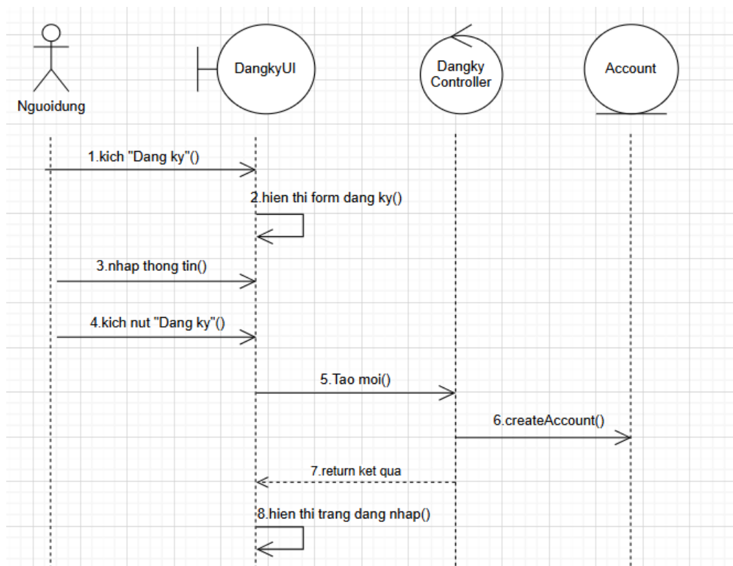
Hình 2.4. Biểu đồ trình tự use case đăng ký
