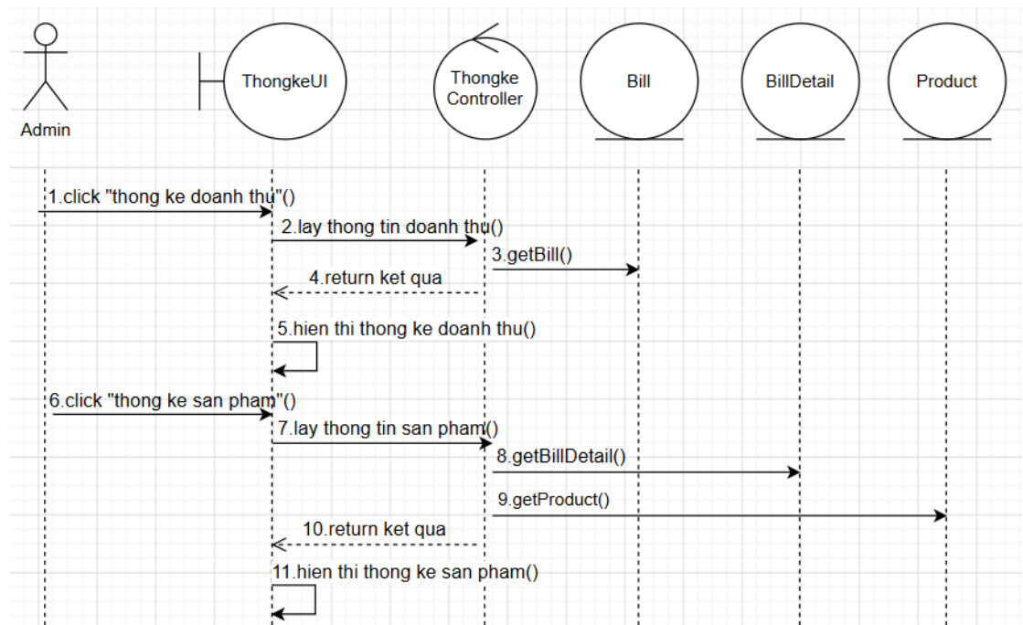
Hình 2.18. Biểu đồ trình tự use case thống kê
