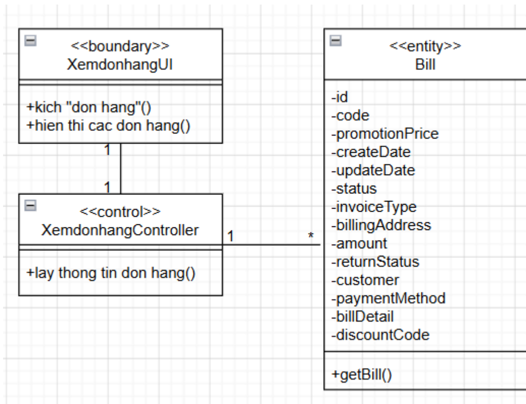
Hình 2.13. Biểu đồ lớp phân tích use case xem lịch sử đơn hàng
