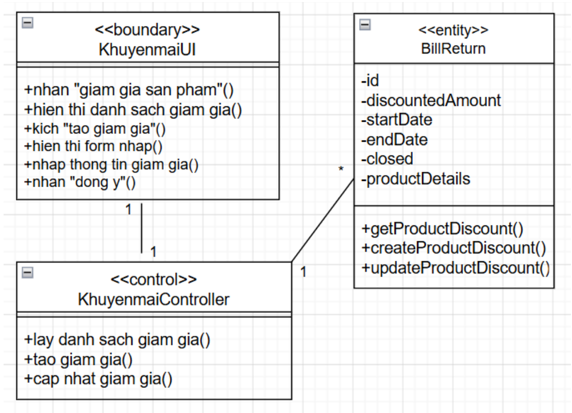
Hình 2.29. Biểu đồ lớp phân tích use case quản lý khuyến mãi sản phẩm
