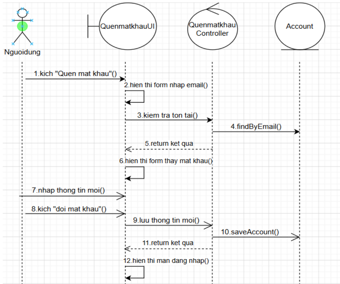
Hình 2.14. Biểu đồ trình tự use case quên mật khẩu
