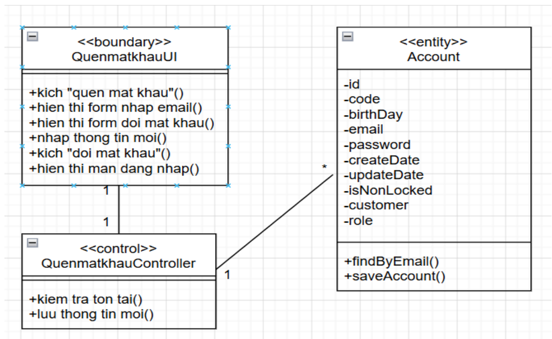
Hình 2.15. Biểu đồ lớp phân tích use case quên mật khẩu
