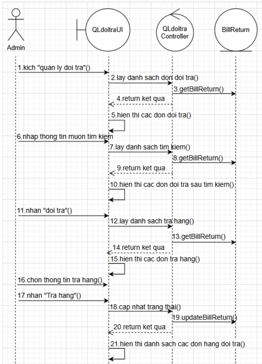
Hình 2.26. Biểu đồ trình tự use case xem quản lý đổi trả
