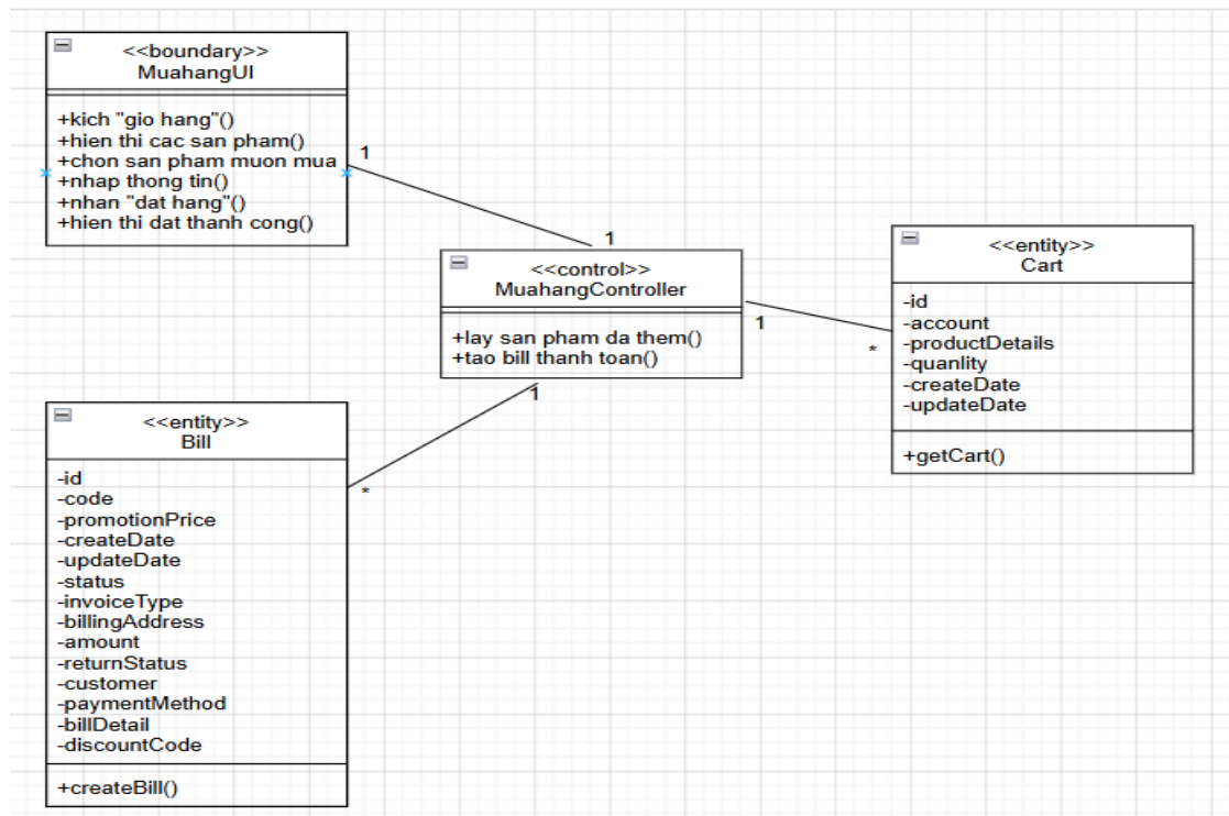
Hình 2.11. Biểu đồ lớp phân tích use case mua hàng
