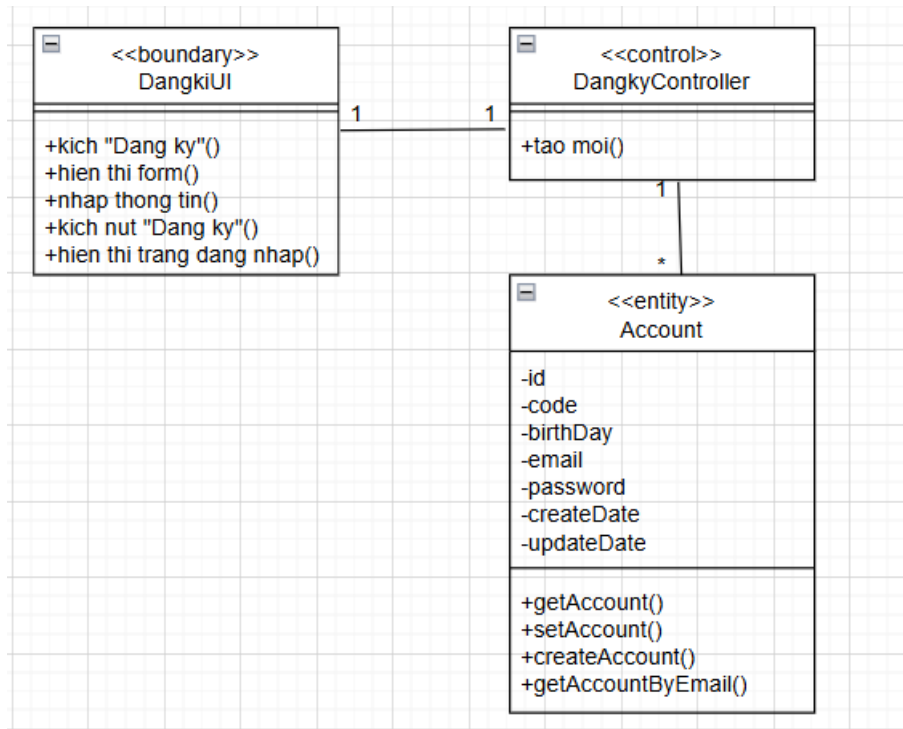
Hình 2.5. Biểu đồ lớp phân tích use case đăng ký
