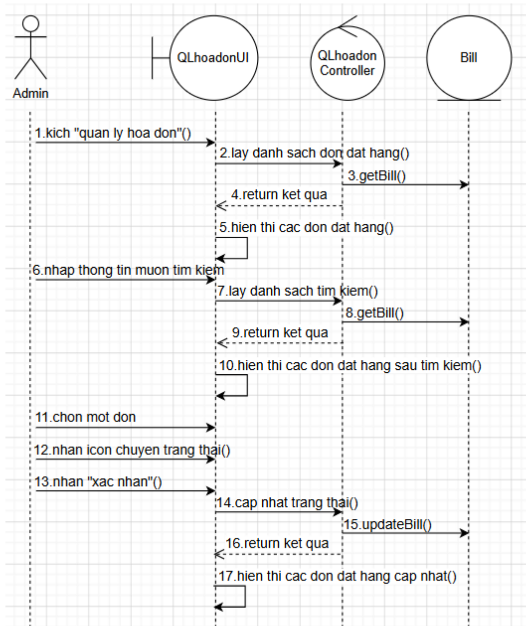
Hình 2.24. Biểu đồ trình tự use case quản lý hóa đơn
