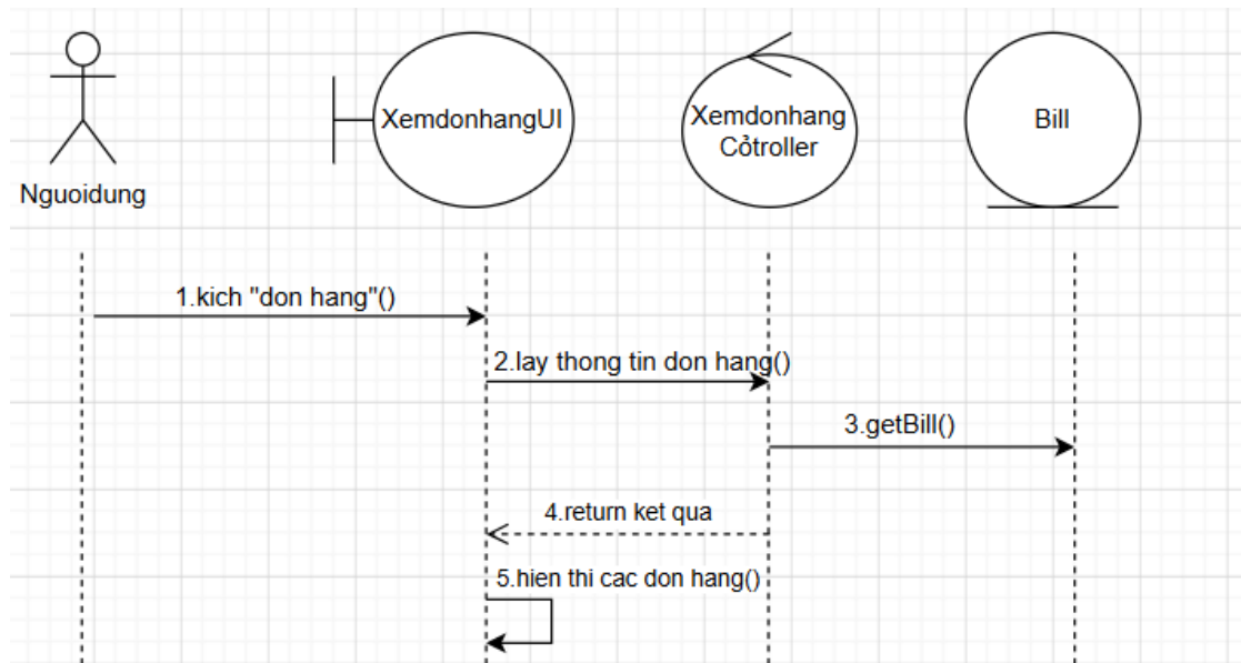
Hình 2.12. Biểu đồ trình tự use case xem lịch sử đơn hàng
