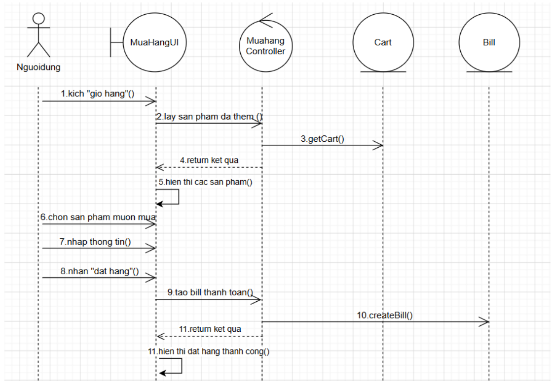
Hình 2.10. Biểu đồ trình tự use case mua hàng
