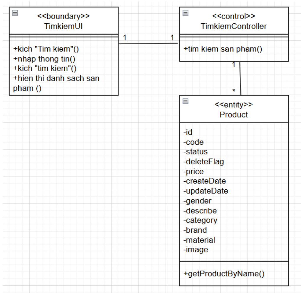
Hình 2.9. Biểu đồ lớp phân tích use case tìm kiếm sản phẩm
