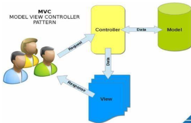
Hình 1.1. Mô hình MVC
