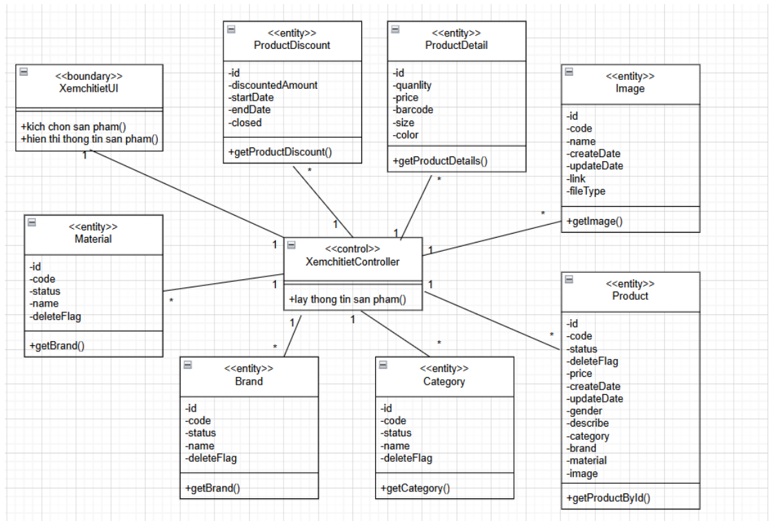
Hình 2.7. Biểu đồ lớp phân tích use case xem chi tiết sản phẩm
