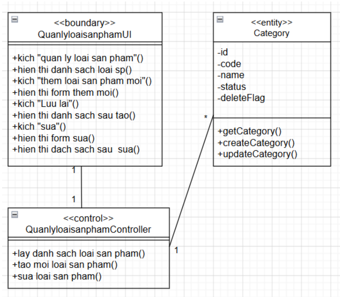
Hình 2.31. Biểu đồ lớp phân tích use case quản lý loại sản phẩm
