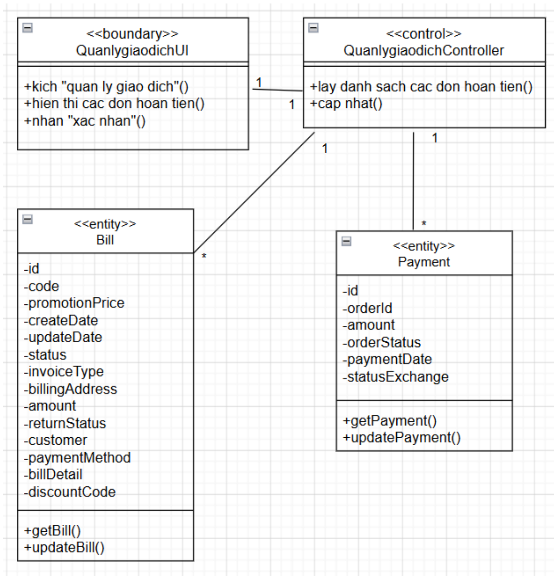
Hình 2.23. Biểu đồ lớp phân tích use case quản lý giao dịch
