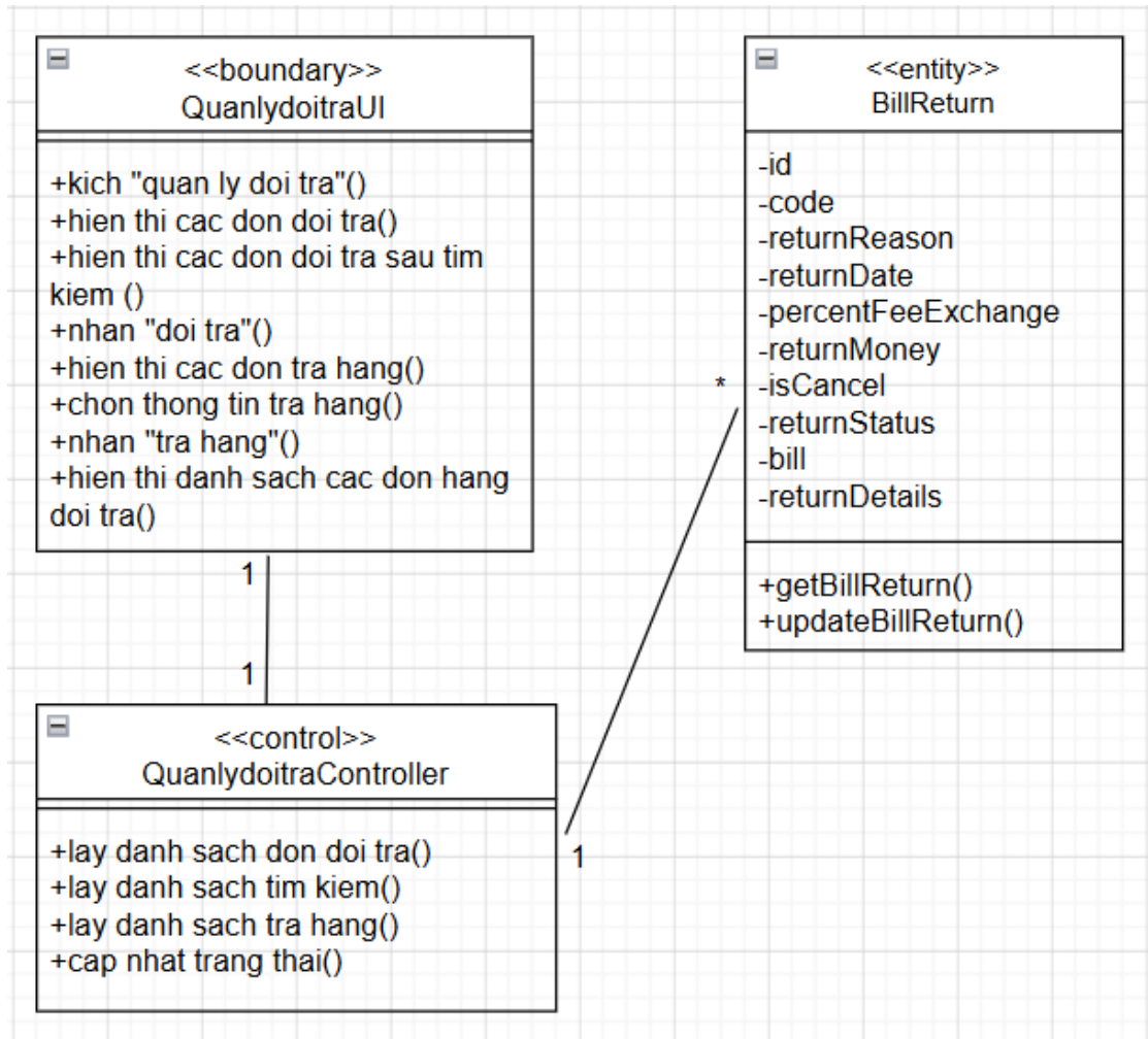
Hình 2.27. Biểu đồ lớp phân tích use case quản lý đổi trả
