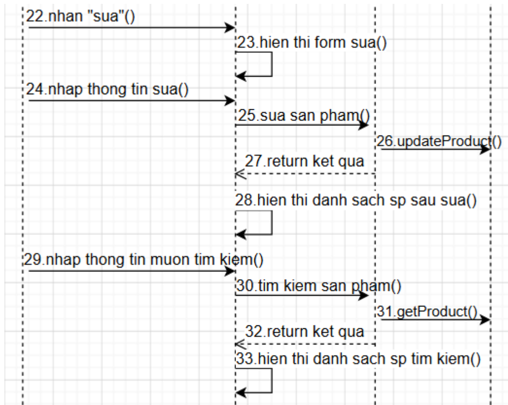
Hình 2.32. Biểu đồ trình tự use case quản lý sản phẩm
