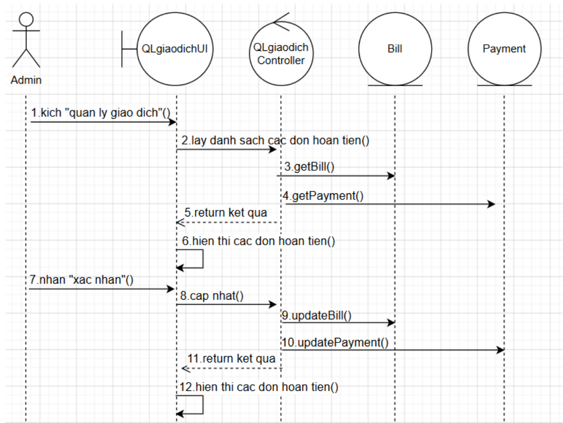
Hình 2.22. Biểu đồ trình tự use case quản lý giao dịch
