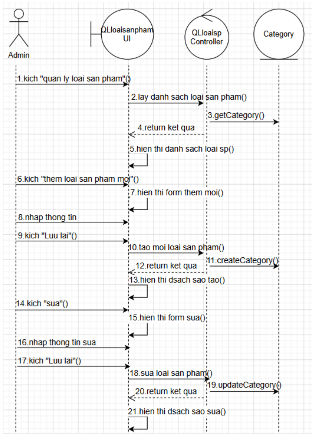
Hình 2.30. Biểu đồ trình tự use case quản lý loại sản phẩm
