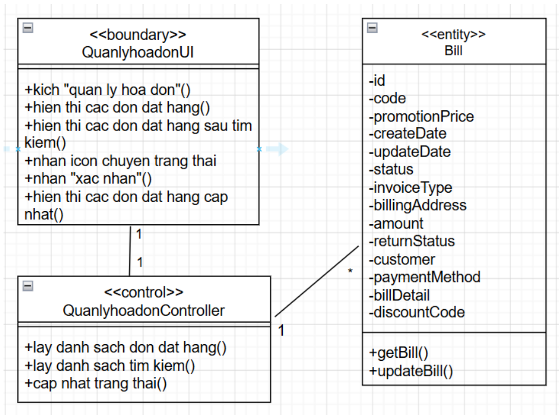
Hình 2.25. Biểu đồ lớp phân tích use case quản lý hóa đơn
