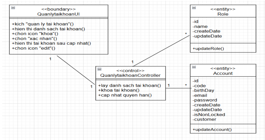
Hình 2.21. Biểu đồ lớp phân tích use case quản lý tài khoản
