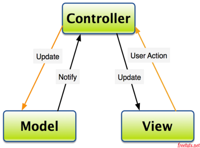
Hình 1.2. Sự tương tác giữa các thành phần trong MVC
