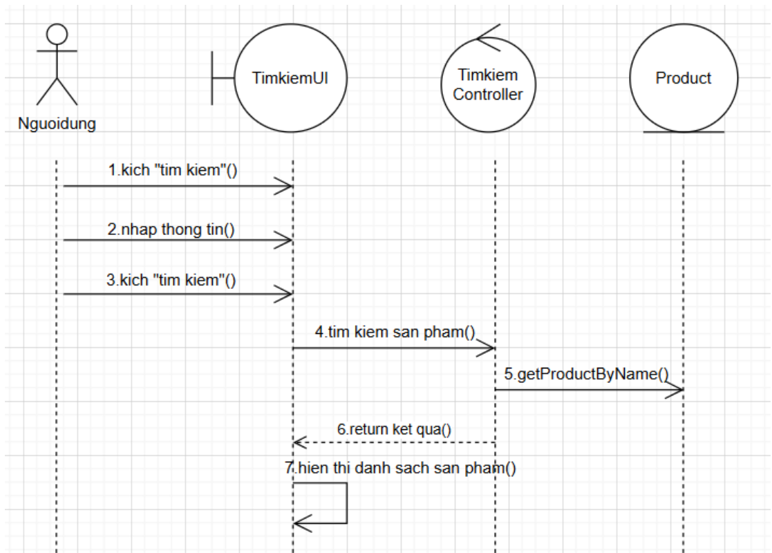
Hình 2.8. Biểu đồ trình tự use case tìm kiếm sản phẩm
