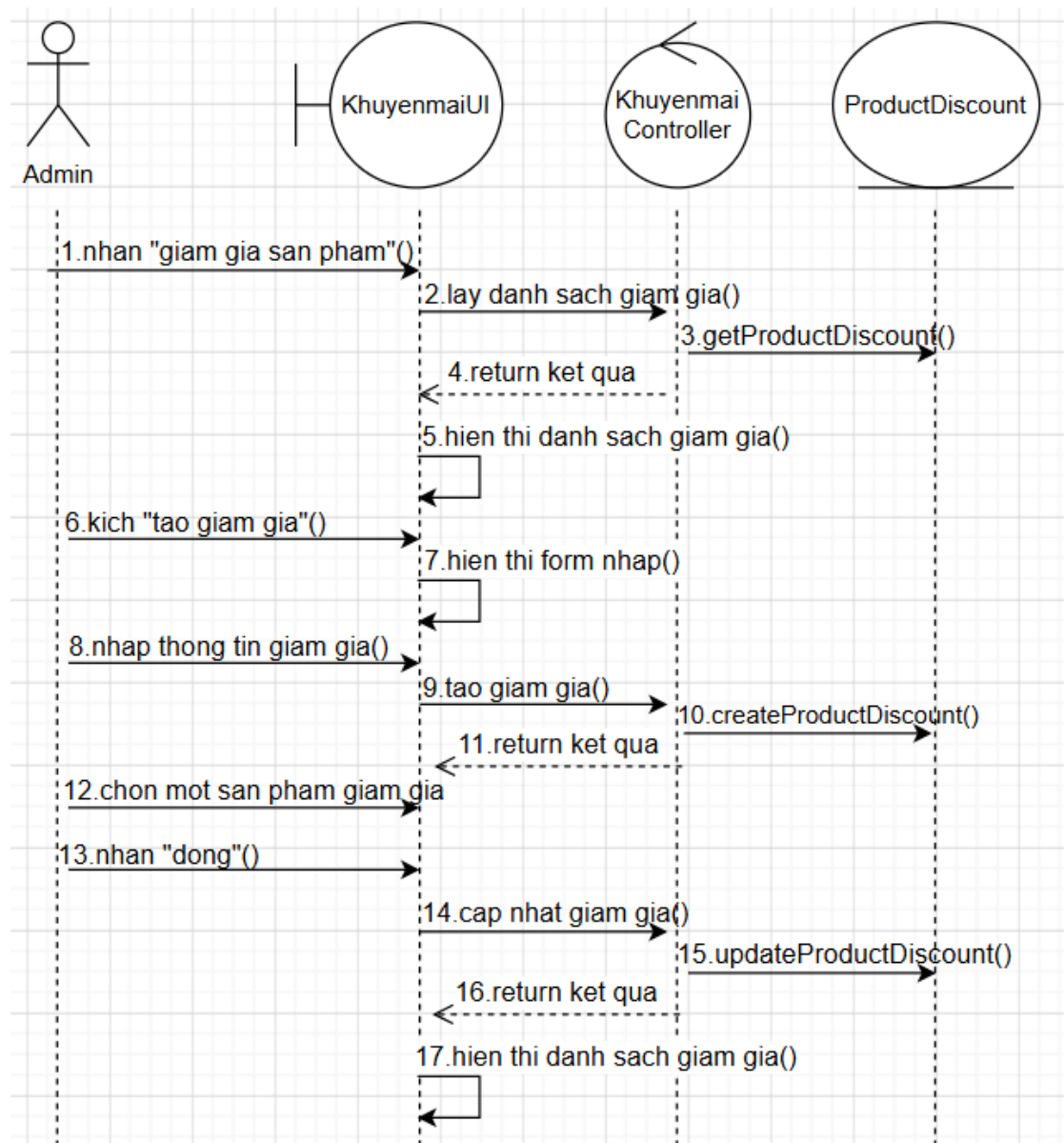
Hình 2.28. Biểu đồ trình tự use case quản lý khuyến mãi sản phẩm
