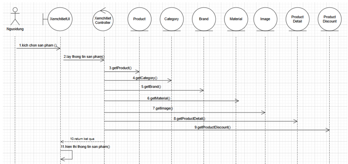
Hình 2.6. Biểu đồ trình tự use case xem chi tiết sản phẩm
