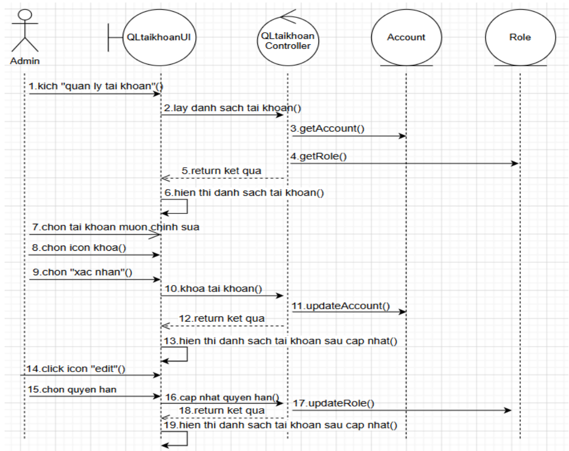
Hình 2.20. Biểu đồ trình tự use case quản lý tài khoản
