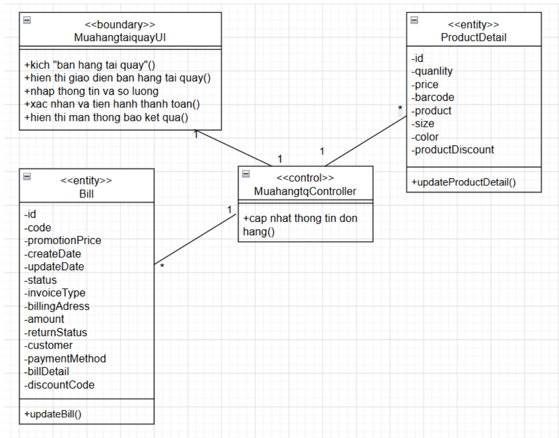
Hình 2.17. Biểu đồ lớp phân tích use case bán hàng tại quầy
