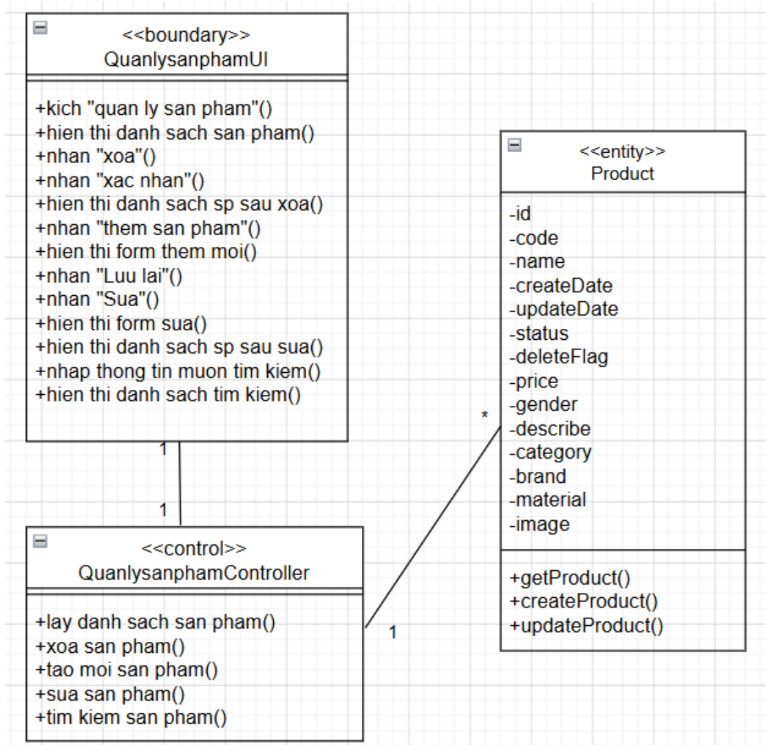
Hình 2.33. Biểu đồ lớp phân tích use case quản lý sản phẩm
