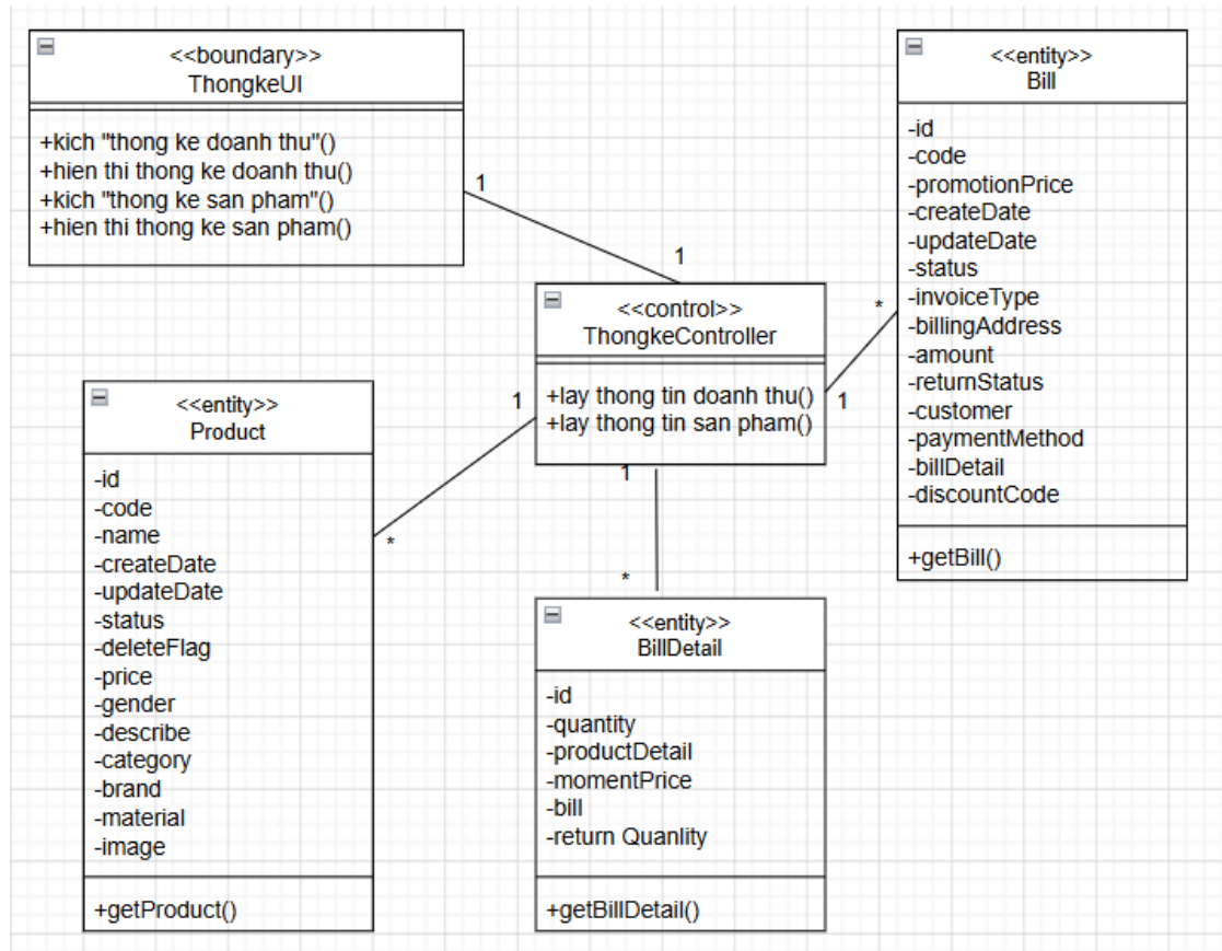
Hình 2.19. Biểu đồ lớp phân tích use case thống kê
