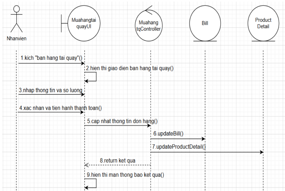
Hình 2.16. Biểu đồ trình tự use case bán hàng tại quầy
