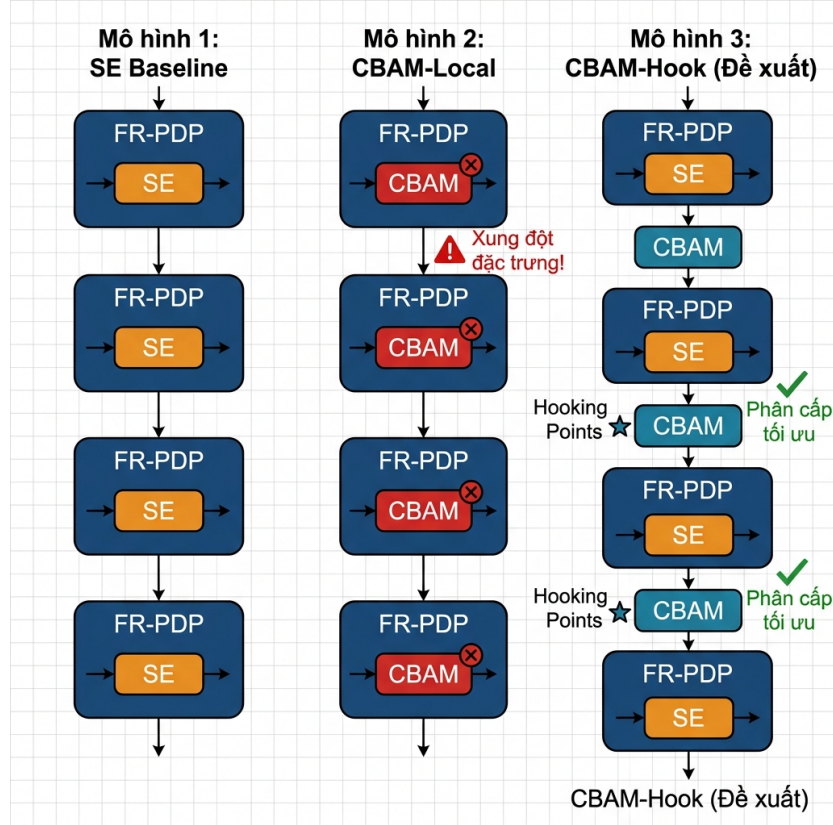
Figure 6: So sánh ba chiến lược: (a) SE Baseline — chỉ SE nội khối, (b) CBAM-Local — thay SE bằng CBAM, gây xung đột, (c) CBAM-Hook — giữ SE, chèn CBAM phân cấp tại điểm nối
