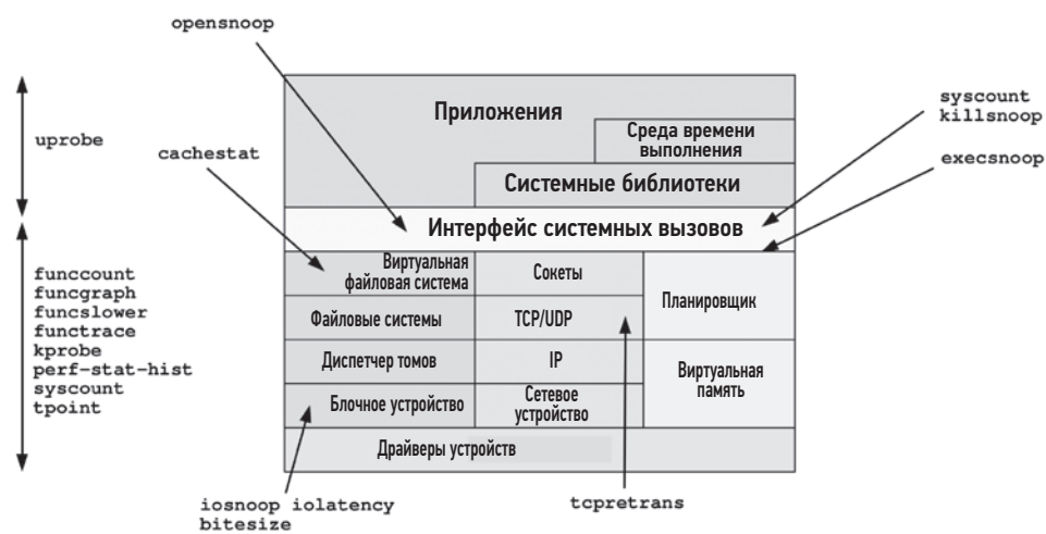
Рис. 14.4. perf-tools
