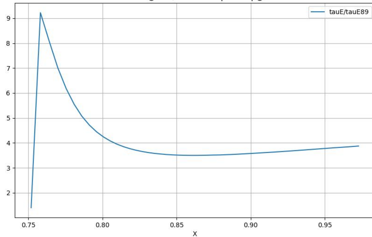
Title: @tauE/tauE89 vs eps*betap@
