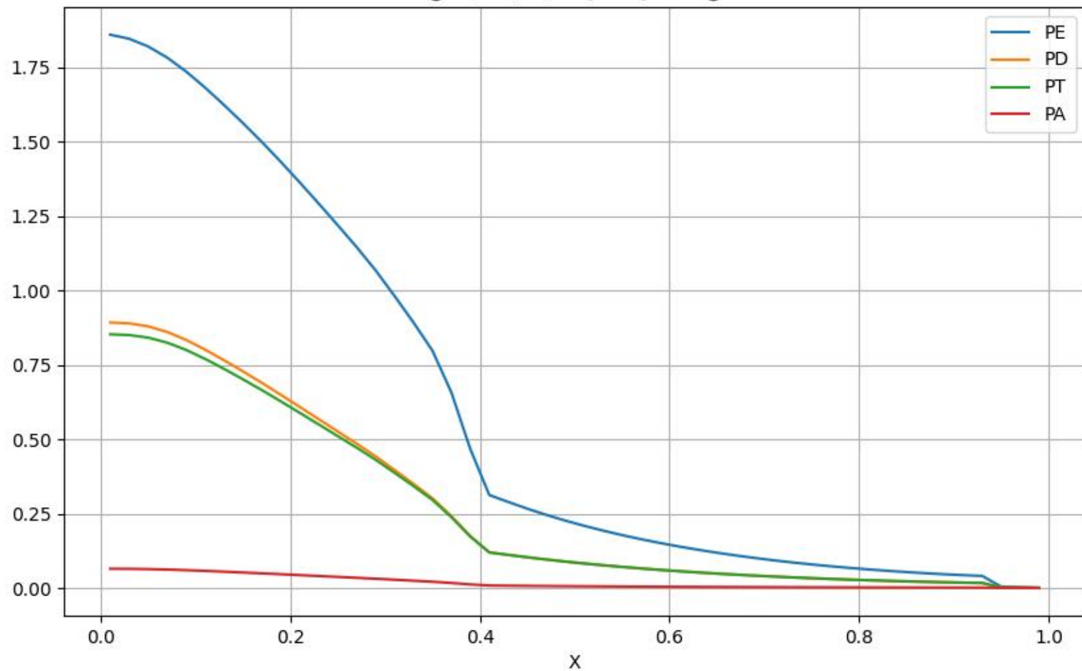
@PE,PD,PT,PA [MPa] vs r@
