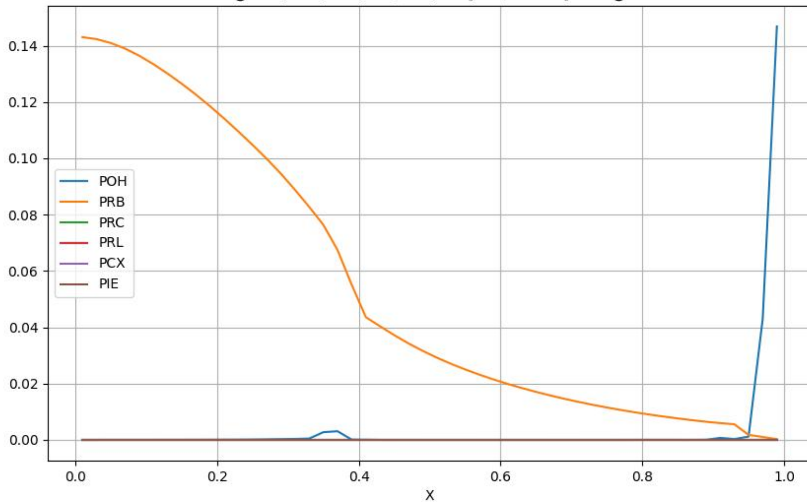
@POH,PRB,PRC,PRL,PCX,PIE [MW/m+3=] vs r@
