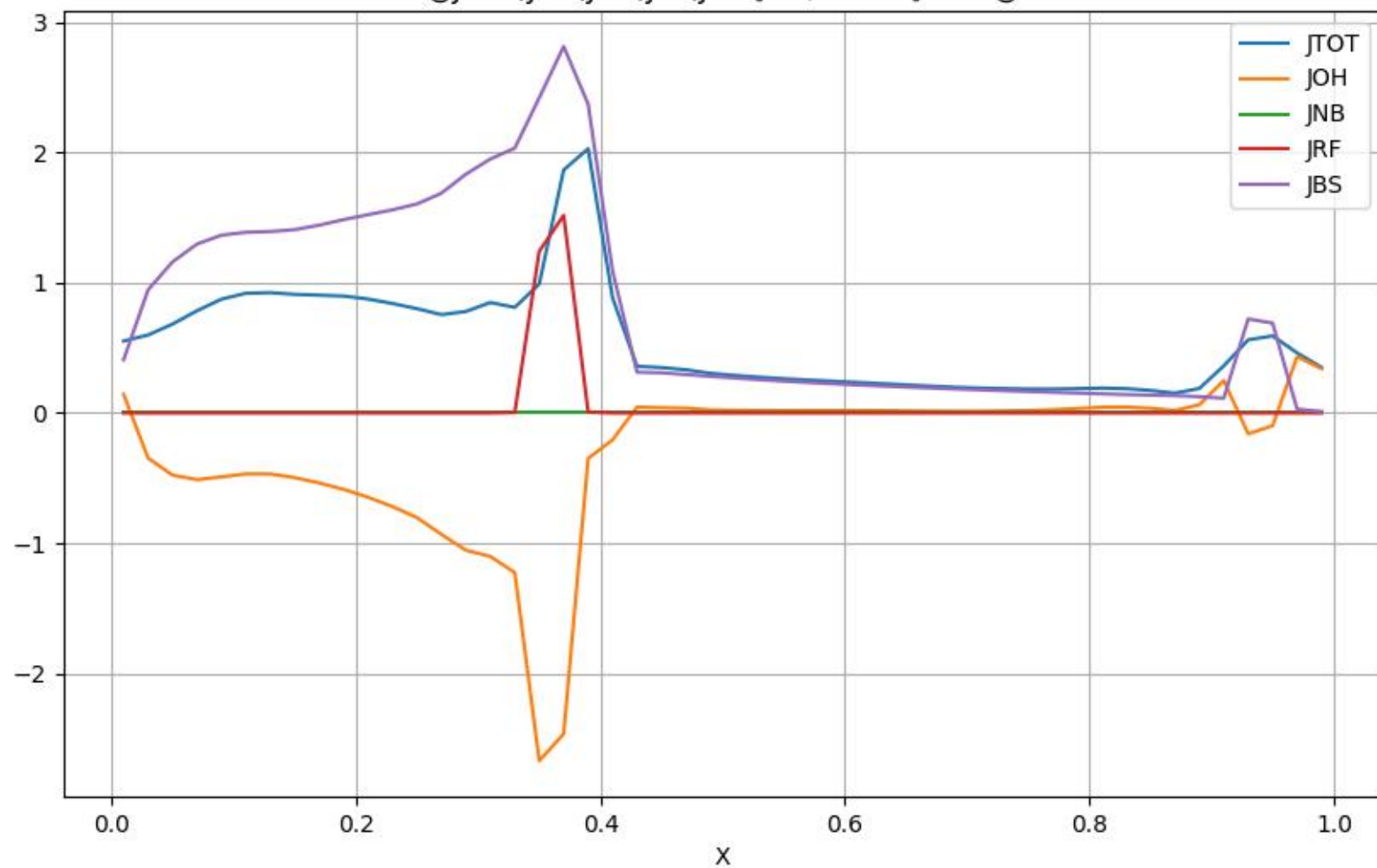
@JTOT,JOH,JNB,JRF,JBS [MA/m+2=] vs r@
