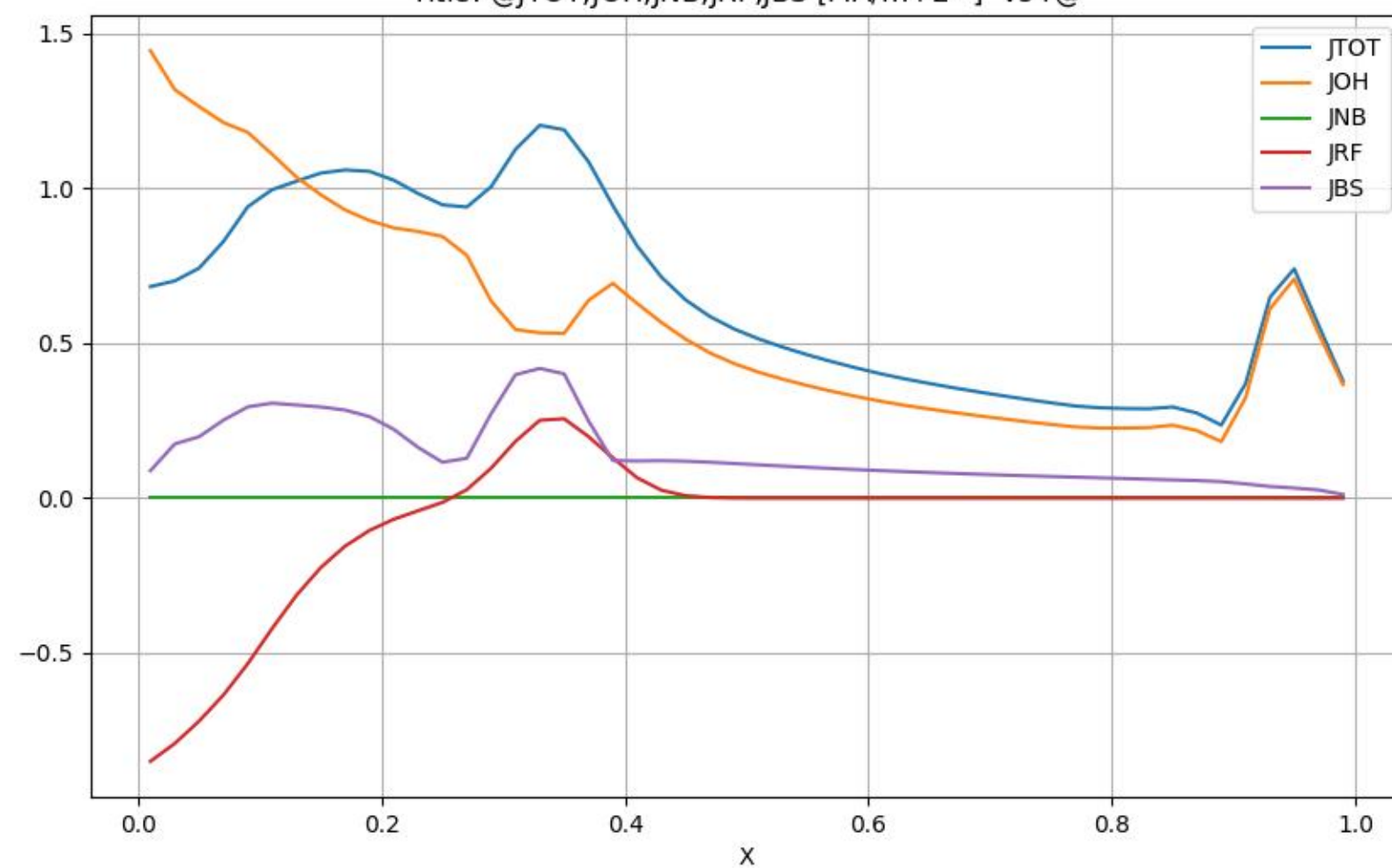
Title: @JTOT,JOH,JNB,JRF,JBS [MA/m+2=] vs r@
