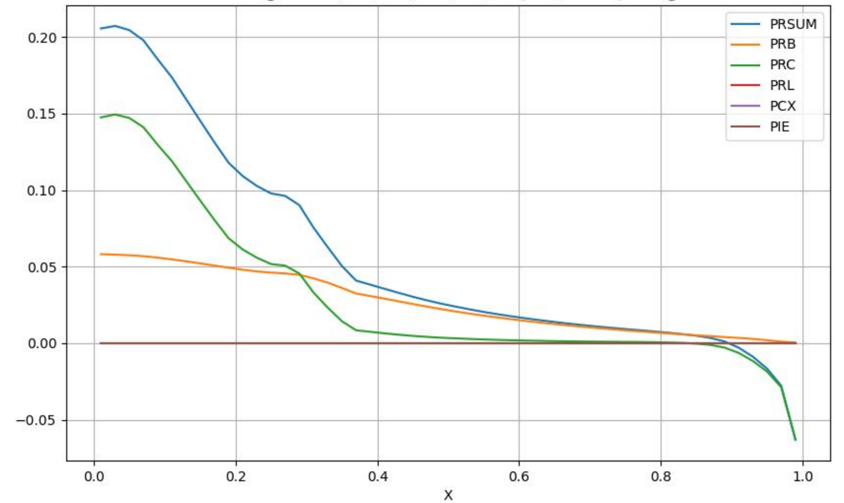
Title: @PRSUM,PRB,PRC,PRL,PCX,PIE [MW/m+3=] vs r@
