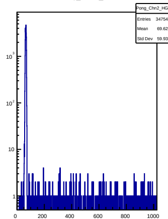
Pong_Chn2_HG
