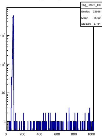
Ping_Chnl21_HG
