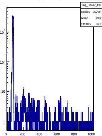
Ping_Chnl7_HG
