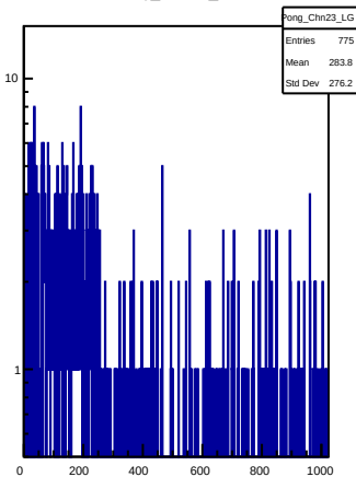
Pong_Chn23_LG
