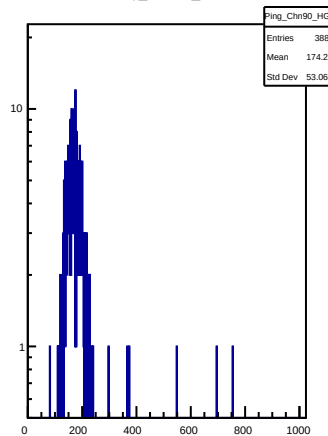
Ping_Chn90_HG
