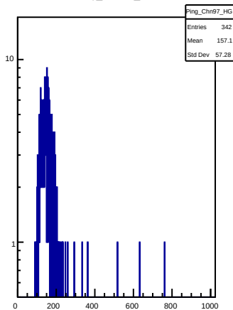
Ping_Ch97_HG
