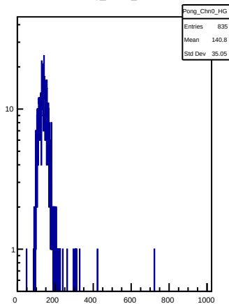
Pong_Chn0_HG
