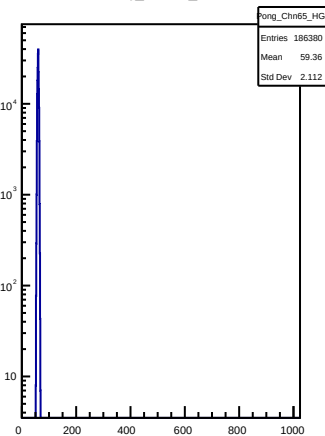
Pong_Chn65_HG
