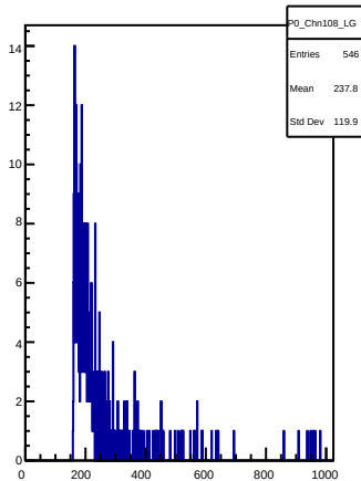
P0_Chnn108_LG
