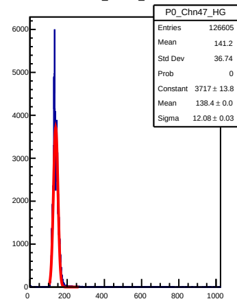
P0_Chn47_HG
