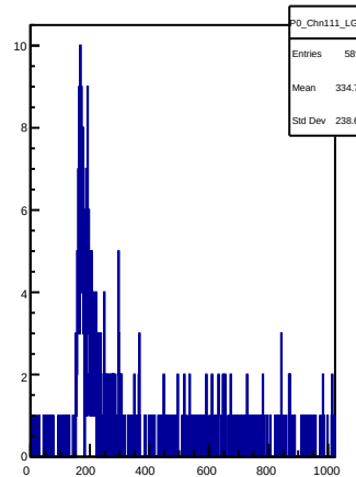
P0_Chnn111_LG
