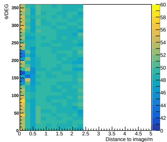
R=[29.1,29.5)\theta=[0.0,10.0)
