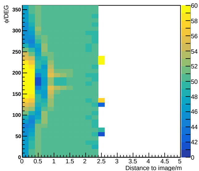
R=[23.8,24.5)\theta=[30.0,40.0)
