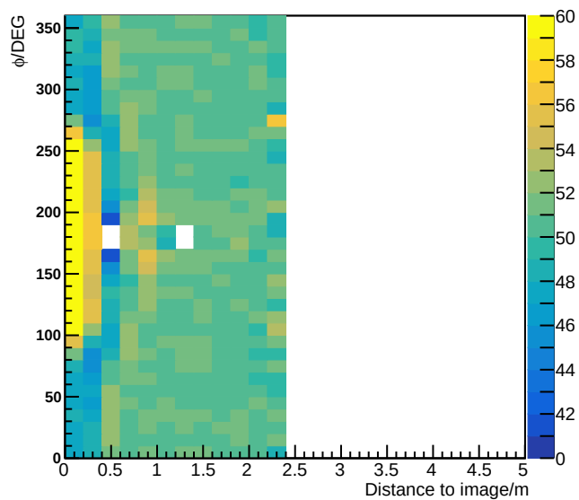
R=[28.1,28.6)\theta=[30.0,40.0)
