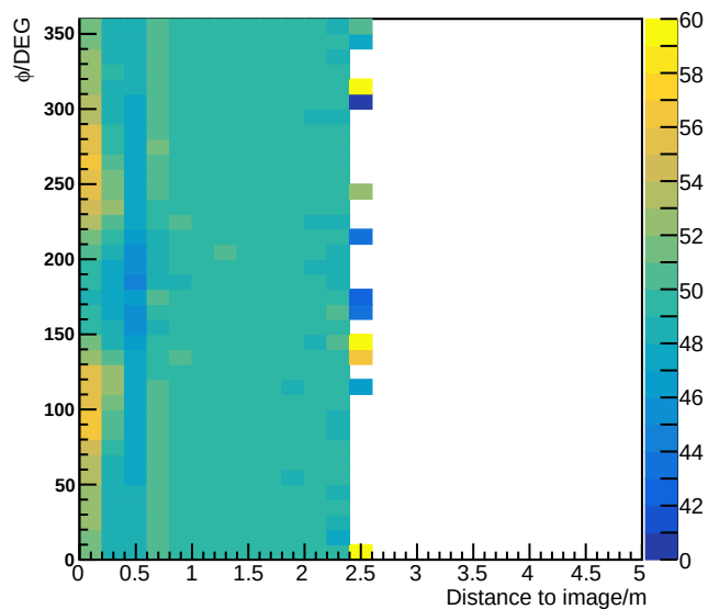
R=[25.2,25.8)\theta=[10.0,20.0)
