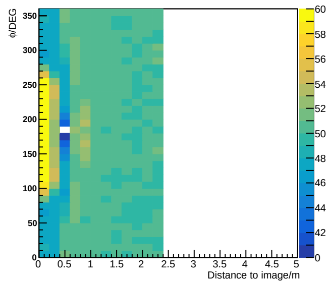
R=[27.0,27.5)\theta=[20.0,30.0)
