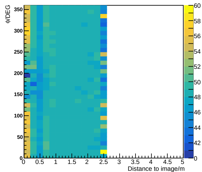
R=[21.4,22.3)\theta=[0.0,10.0)
