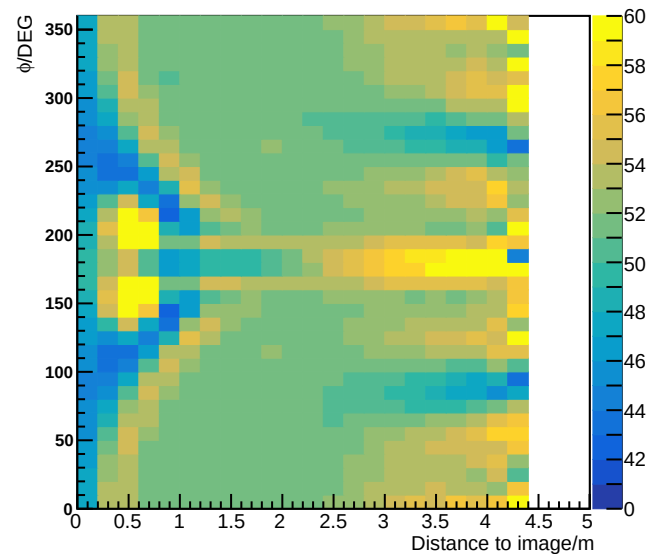
R=[3.9,10.9)\theta=[40.0,50.0)
