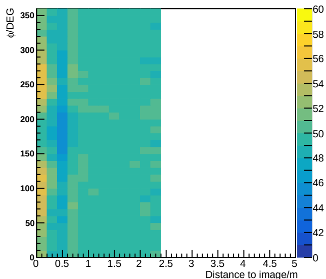
R=[29.5,30.0)\theta=[10.0,20.0)
