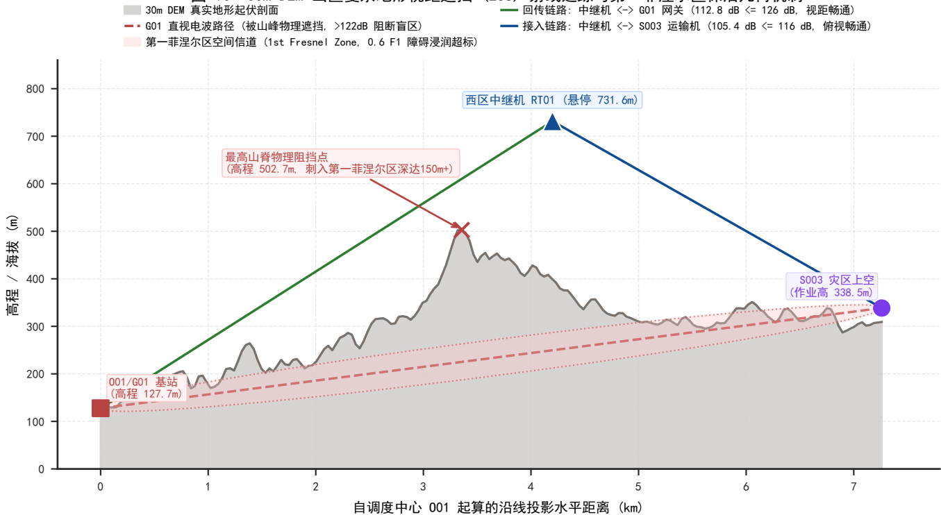
图 10 30m DEM 山区复杂地形视距遮挡 (LOS) 射线追踪与第一菲涅尔区保活几何机制
