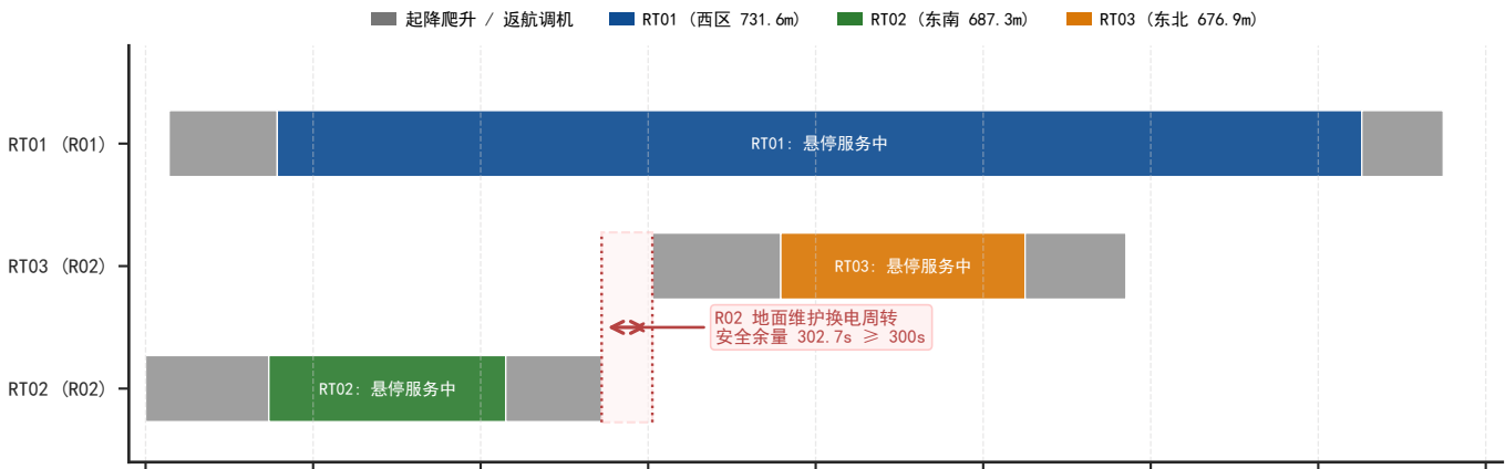
(a) 中继无人机执飞架次空间部署与时空覆盖甘特图
