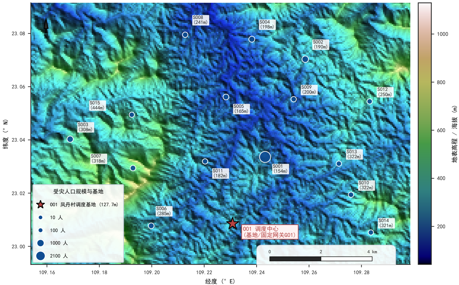
图 1 广西横州镇龙乡高精度 30m DEM 地貌阴影晕渲与应急救援网络拓扑
