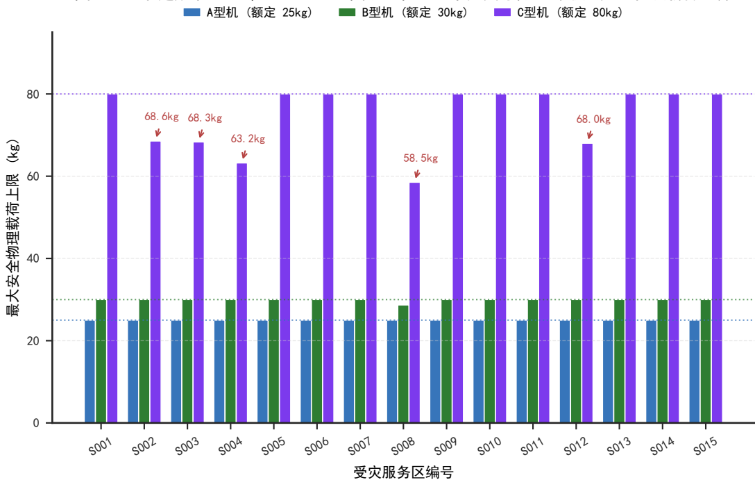
图 4 基准返航余量 ( \eta=0.20 ) 下三类机型在 15 个受灾服务区的最大安全物理载荷上限
