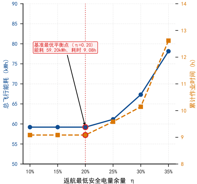
(b) 能耗与耗时随电量余量剧增的临界相变
