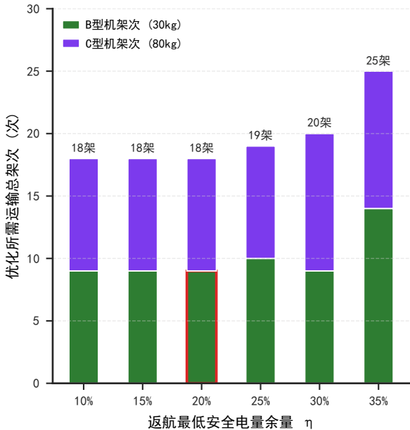
(a) 安全电量余量 \eta 对总架次及机型构成的影响
