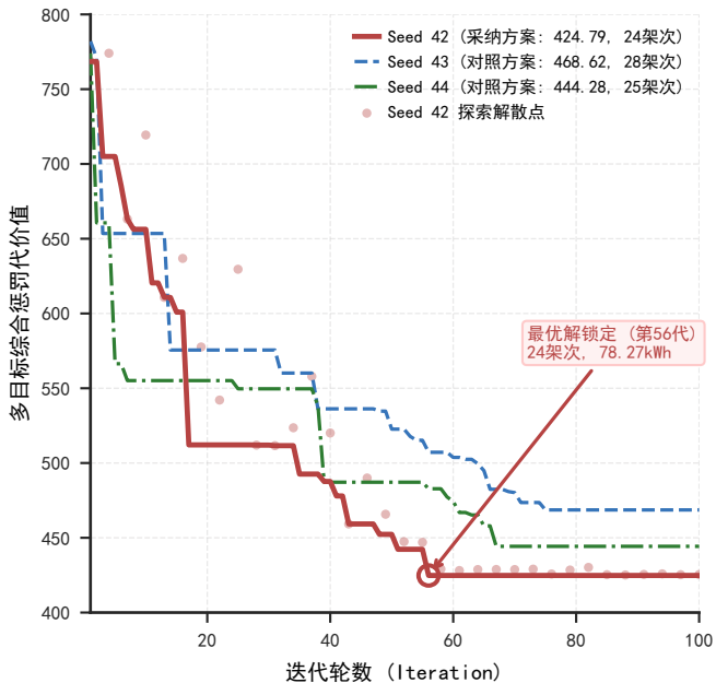
(a) ALNS 启发式算法 100 代阶梯收敛轨迹 (真实日志)
