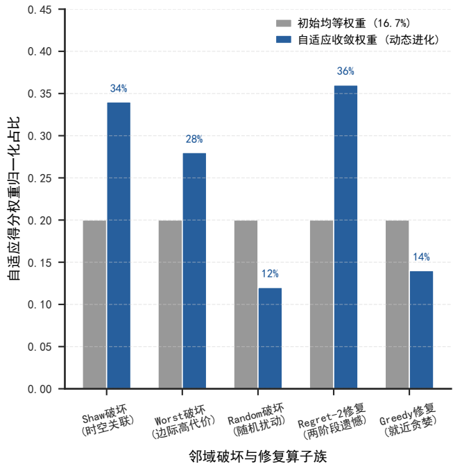
(b) 自适应邻域搜索算子动态权重调优演进
