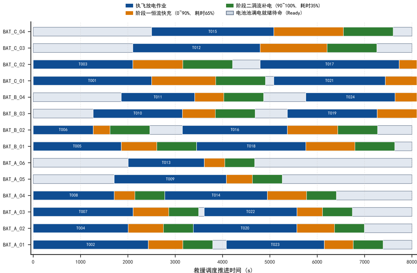
图 8 14 组共享电池车电分离两阶段等效电流流水线推进全景 (0 冲突周转)
