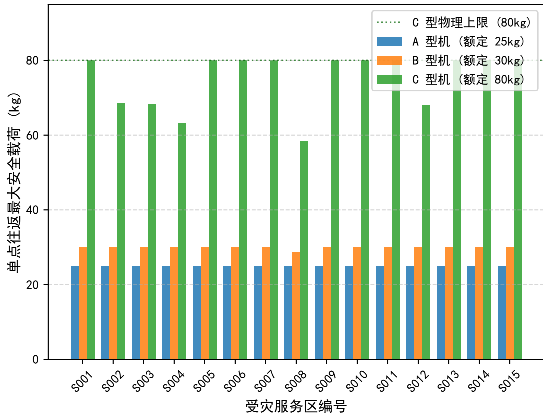
(a) 各机型在各服务区单点往返最大安全载重量
