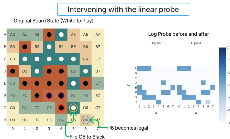
Hình 7.6: Nghiên cứu Othello-GPT cho thấy một mô hình Transformer, chỉ được huấn luyện trên chuỗi nước đi, đã tự học cách biểu diễn trạng thái của bàn cờ bên trong nó.
