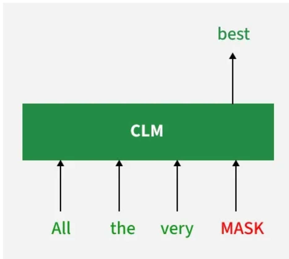
Hình 4.5: Mục tiêu huấn luyện của GPT: Causal Language Modeling. Tại mỗi bước, mô hình cố gắng dự đoán từ tiếp theo dựa trên các từ trước đó.
