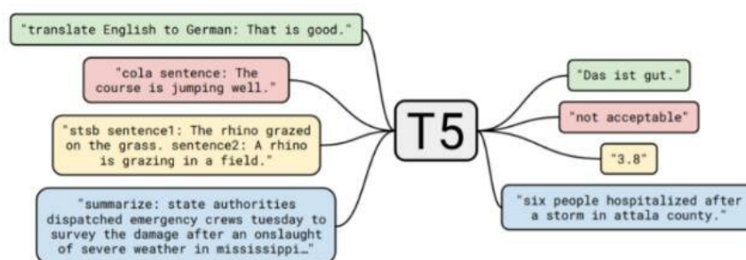
Hình 4.7: Khung “Text-to-Text” của T5: mọi tác vụ đều được biểu diễn dưới dạng chuỗi vào–ra.
