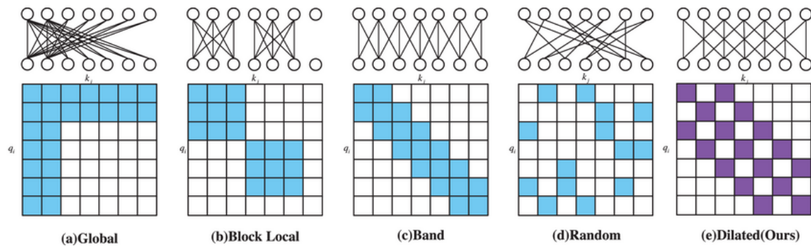
Hình 4.8: So sánh các mẫu chú ý thưa (sparse attention). (a) Chú ý toàn cục (Global). (b) Chú ý theo khối cục bộ (Block Local). (c) Chú ý theo dải (Band), hay còn gọi là cửa sổ trượt (Sliding Window). (d) Chú ý ngẫu nhiên (Random). (e) Chú ý giãn cách (Dilated). Các mô hình như Longformer và BigBird thường kết hợp các mẫu này.
