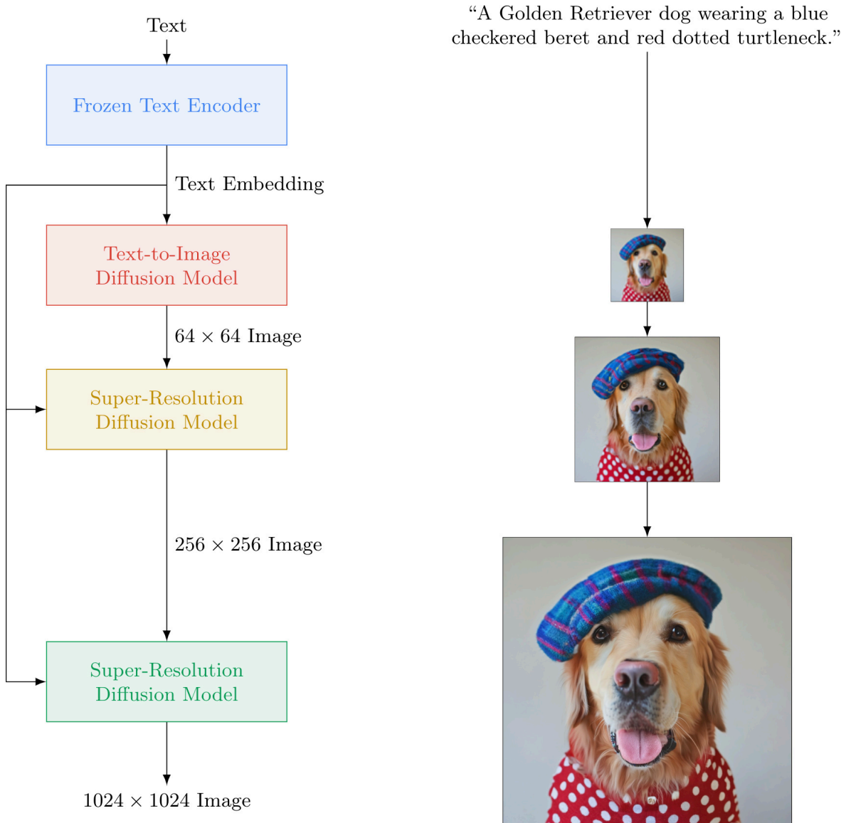
Hình 7.5: Mô hình Khuếch tán cho việc sinh ảnh từ văn bản. Bắt đầu từ nhiễu, mô hình dần dần khử nhiễu theo sự dẫn dắt của embedding văn bản để tạo ra ảnh cuối cùng.
