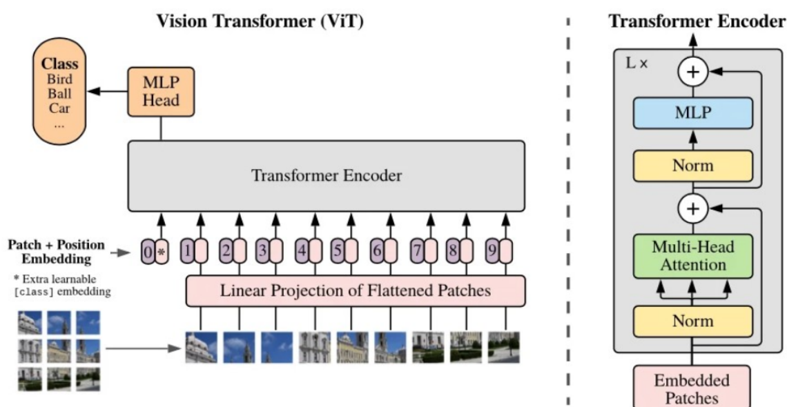
Hình 7.3: Kiến trúc của Vision Transformer (ViT). Ảnh được chia thành các mảnh vâ, mỗi mảnh được nhúng và xử lý như một "token" trong một chuỗi bởi một Transformer Encoder tiêu chuẩn.
