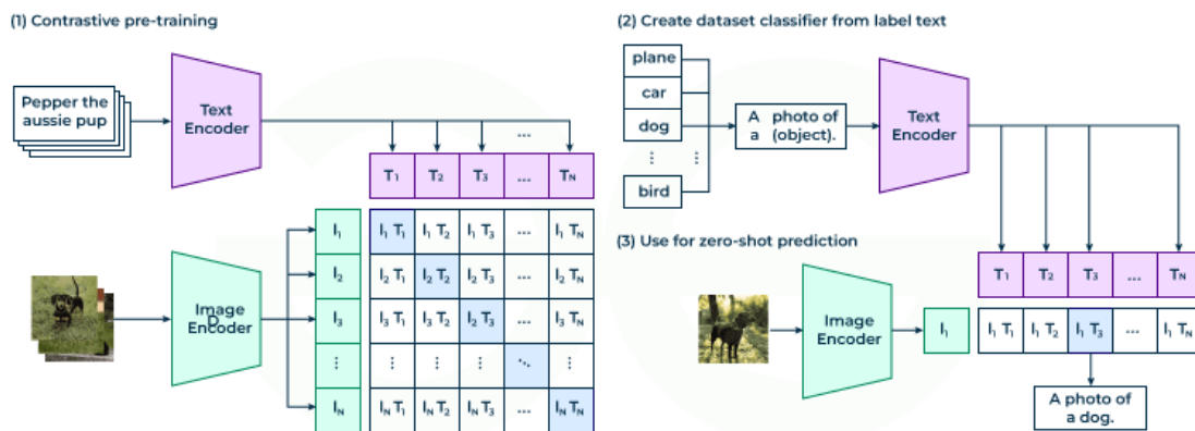
Hình 7.4: Quy trình huấn luyện của CLIP. Mô hình học cách tối đa hóa độ tương đồng của các cặp (ảnh, văn bản) chính xác trên đường chéo chính và tối thiểu hóa độ tương đồng của các cặp không chính xác.
