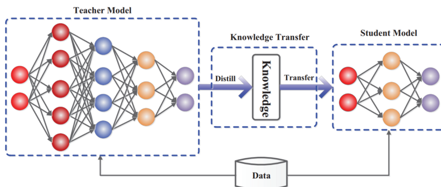
Hình 7.1: Quy trình Chung cất Tri thức. Mô hình trò học đồng thời từ nhãn cứng của dữ liệu (Hard Loss) và nhãn mềm được tạo ra bởi mô hình thầy (Soft Loss).
