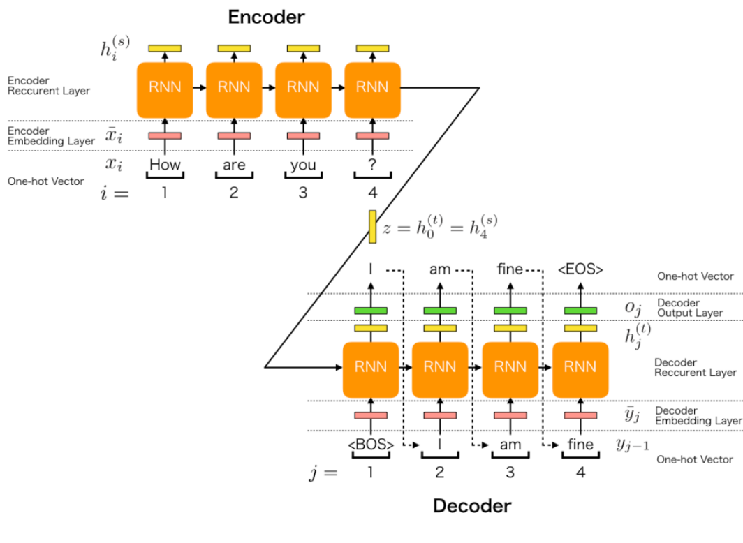
Hình 3.6: Kiến trúc Encoder-Decoder tổng quát. Encoder ”đọc” và nén chuỗi đầu vào thành một vector ngữ cảnh. Decoder sử dụng vector này để ”viết” ra chuỗi đầu ra.
