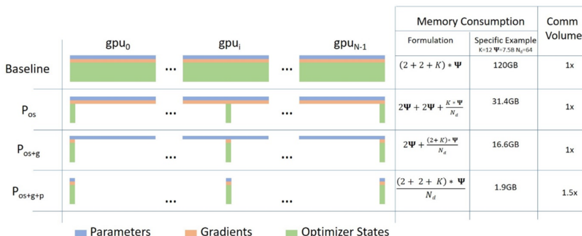
Hình 2.3: So sánh việc sử dụng bộ nhớ trong Data Parallelism tiêu chuẩn và các giai đoạn của ZeRO. ZeRO giảm đáng kể sự thừa thãi bằng cách phân mảnh các thành phần của quá trình huấn luyện.
