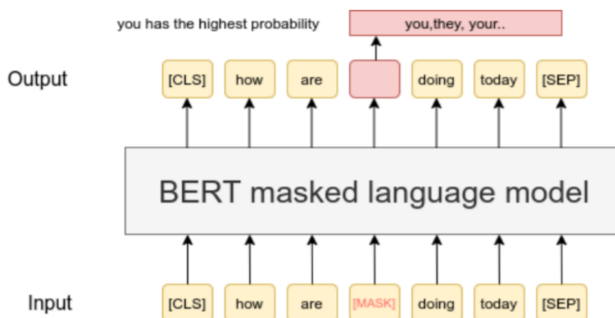
Hình 4.3: Mục tiêu huấn luyện kinh điển của BERT: Masked Language Modeling (MLM). Mô hình phải dự đoán các token bị che dựa trên ngữ cảnh hai chiều.
