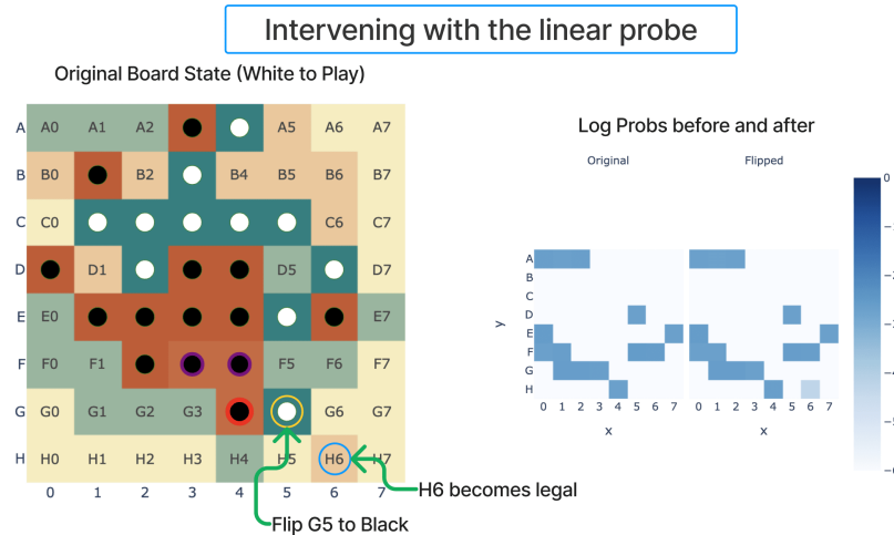
Hình 6.7: Nghiên cứu Othello-GPT cho thấy một mô hình Transformer, chỉ được huấn luyện trên chuỗi nước đi, đã tự học cách biểu diễn trạng thái của bàn cờ bên trong nó.
