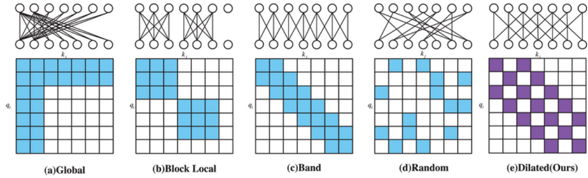
Hình 4.5: So sánh các mẫu chú ý thưa (sparse attention). (a) Chú ý toàn cục (Global). (b) Chú ý theo khối cục bộ (Block Local). (c) Chú ý theo dải (Band), hay còn gọi là cửa sổ trượt (Sliding Window). (d) Chú ý ngẫu nhiên (Random). (e) Chú ý giãn cách (Dilated). Các mô hình như Longformer và BigBird thường kết hợp các mẫu này.
