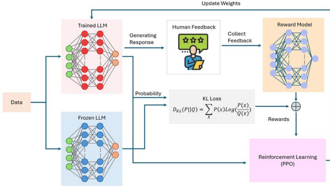
Hình 5.3: Quy trình ba bước của RLHF: (1) Supervised Fine-Tuning (SFT), (2) Reward Model (RM), (3) Policy Optimization (PPO).
