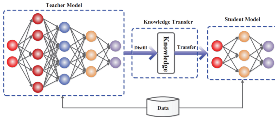
Hình 6.2: Quy trình Chưng cất Tri thức. Mô hình trò học đồng thời từ nhãn cứng của dữ liệu và nhãn mềm (được tạo ra bởi mô hình thầy với hiệu độ T ).
