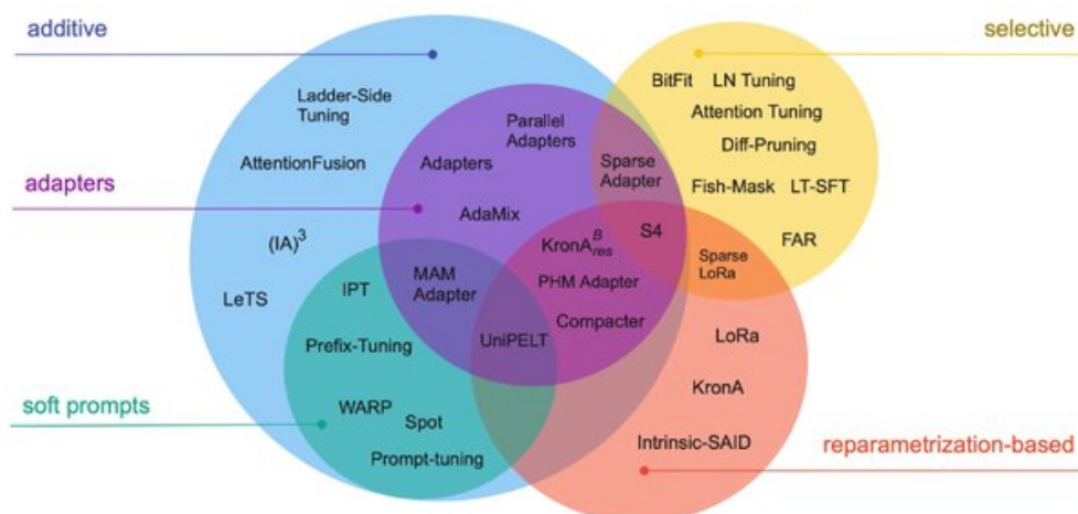
Hình 5.2: Minh họa trực quan: 5 nhóm chính PEFT và các giao nhau (ví dụ tiêu biểu).
