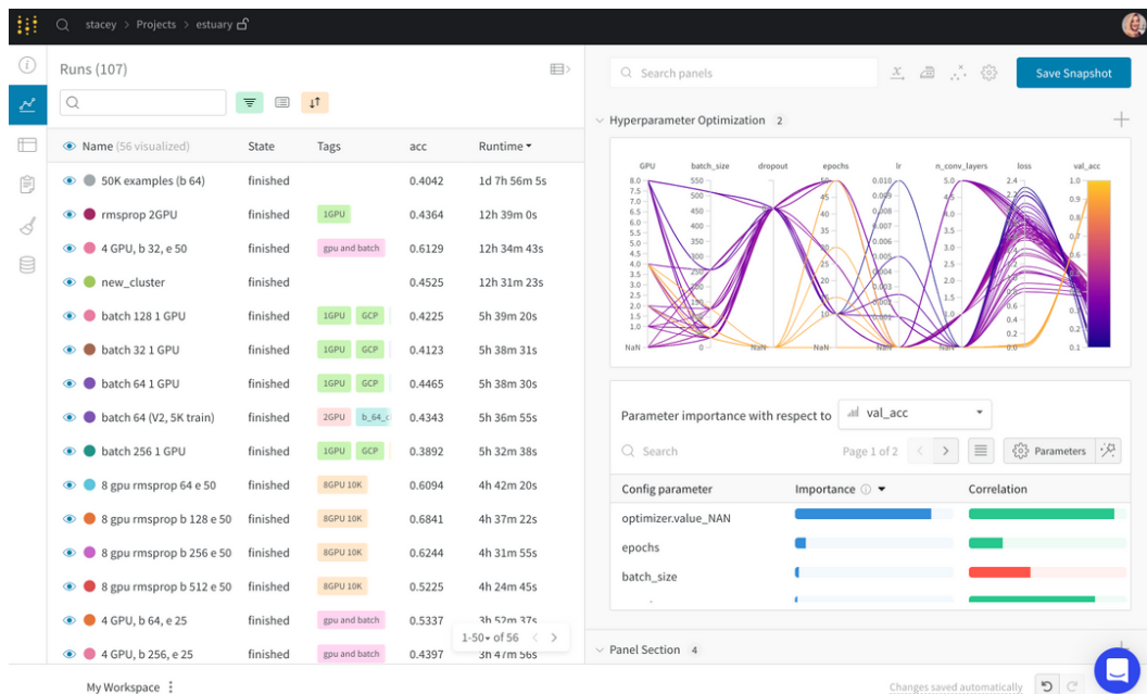
Hình 2.2: Một trang tổng quan (dashboard) điển hình trong Weights & Biases, cho phép so sánh nhiều lần chạy thí nghiệm một cách trực quan.
