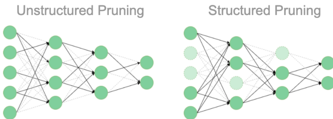
Hình 6.3: So sánh Cắt tỉa Không có Cấu trúc (xóa các trọng số riêng lẻ, tạo ma trận thưa thớt) và Cắt tỉa Có Cấu trúc (xóa toàn bộ cột/nơ-ron, tạo ma trận nhỏ hơn).
