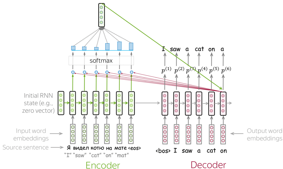
Hình 3.7: Cơ chế Chú ý trong Seq2Seq. Tại bước sinh từ thứ t của Decoder, nó tính toán các trọng số chú ý ( \alpha_t ) để tạo ra một vector ngữ cảnh động ( c_t ) từ tất cả các trạng thái ẩn của Encoder.
