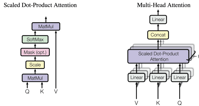
Hình 4.1: Sơ đồ Scaled Dot-Product Attention. Đầu vào là các ma trận Q, K, V và đầu ra là một ma trận đã được làm giàu ngữ cảnh.
