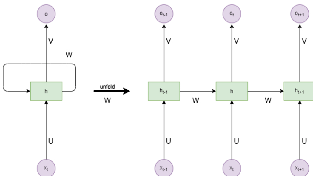
Hình 3.4: Kiến trúc của một RNN. Bên trái là dạng nén với vòng lặp. Bên phải là dạng "trải ra theo thời gian" (unrolled), cho thấy cách trạng thái ẩn h được truyền từ bước này sang bước tiếp theo.
