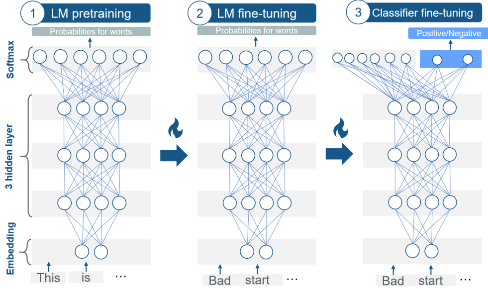
Hình 3.9: Quy trình 3 bước của ULMFiT: Pre-training trên dữ liệu chung, Fine-tuning LM trên dữ liệu miền đích, và Fine-tuning bộ phân loại cho tác vụ cuối cùng.
