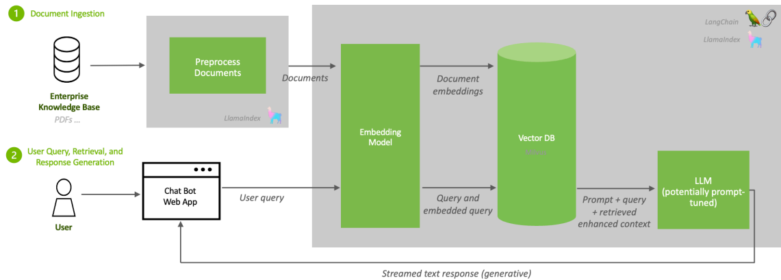
Hình 6.1: Sơ đồ kiến trúc của một hệ thống RAG, bao gồm giai đoạn Lập chỉ mục (bên trên) và giai đoạn Truy vấn (bên dưới).
