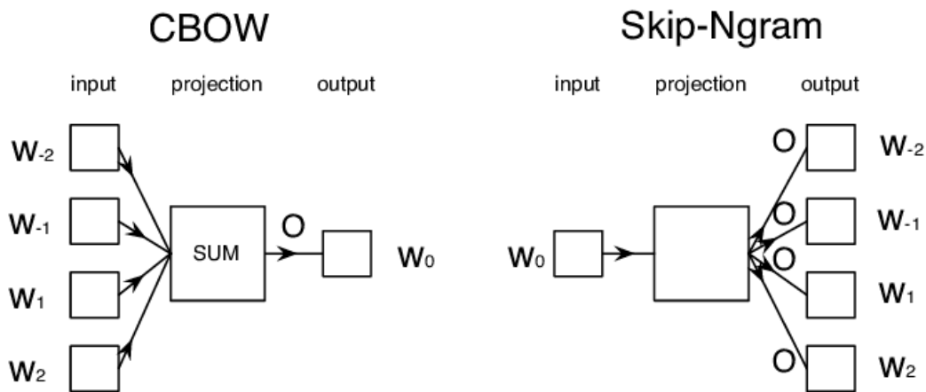
Hình 3.2: So sánh trực quan giữa CBOW (tổng hợp ngữ cảnh để dự đoán 1 từ) và Skip-gram (dùng 1 từ để dự đoán nhiều từ trong ngữ cảnh, tạo thành các cặp huấn luyện riêng biệt).
