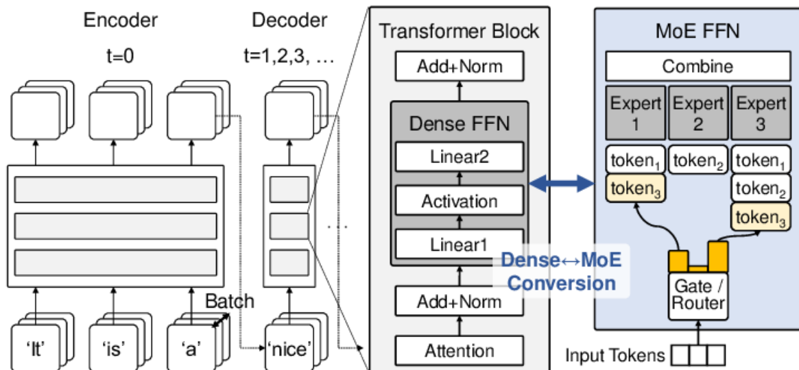
Hình 4.6: So sánh một khối Transformer tiêu chuẩn (trái) và một khối Transformer với lớp MoE (phải). Lớp FFN dày đặc được thay thế bằng một mạng cổng và nhiều chuyên gia FFN thưa thớt.
