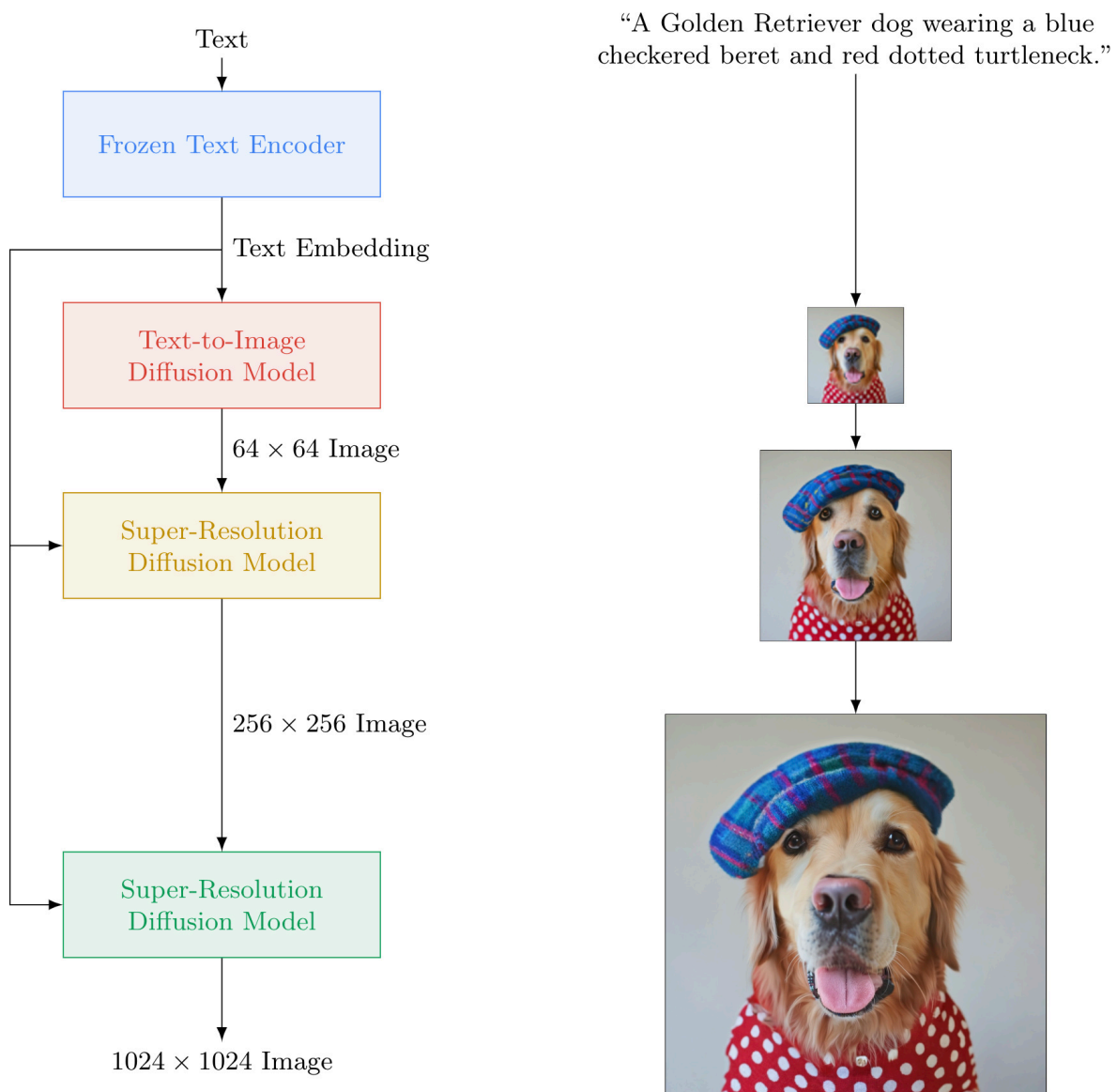
Hình 6.6: Mô hình Khuếch tán cho việc sinh ảnh từ văn bản. Bắt đầu từ nhiễu, mô hình dần dần khử nhiễu theo sự dẫn dắt của embedding văn bản để tạo ra ảnh cuối cùng.
