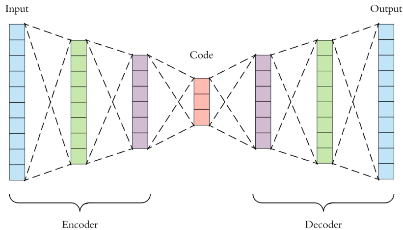
Hình 3.3: Kiến trúc tổng quát của Autoencoder. Phần hẹp nhất ( bottleneck ) chính là không gian ẩn chứa thông tin nén.
