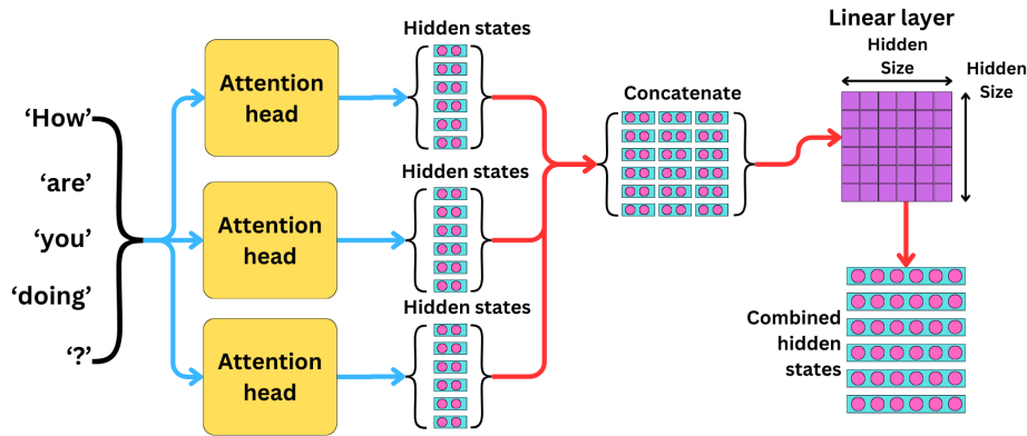
Hình 4.2: Kiến trúc Multi-Head Attention, bao gồm nhiều "đầu" Scaled Dot-Product Attention chạy song song.
