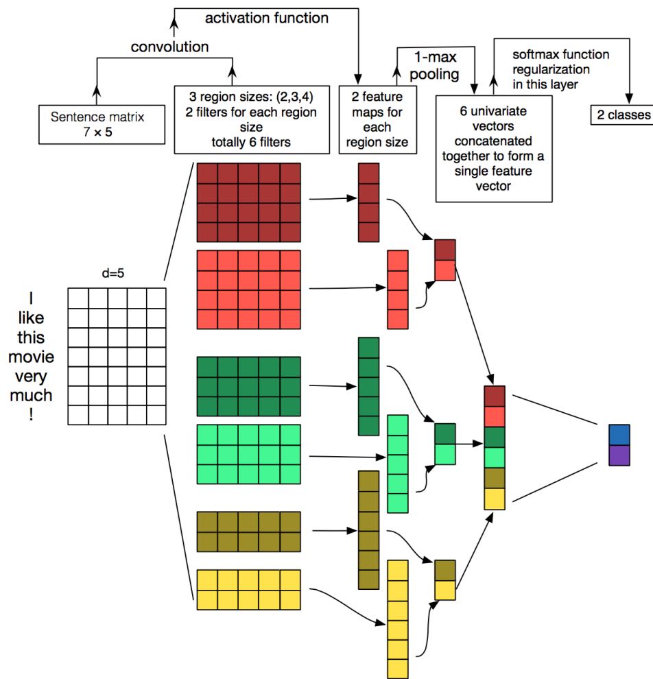
Hình 3.8: Kiến trúc CNN cho phân loại văn bản. Các bộ lọc có kích thước khác nhau (2, 3, 4 từ) trượt dọc theo câu để trích xuất các đặc trưng N-gram. Kết quả sau đó được gộp lại (max-pooling) và đưa vào một lớp FNN để phân loại.
