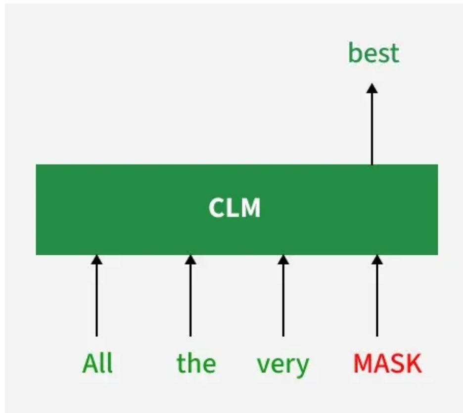
Hình 4.4: Mục tiêu huấn luyện của GPT: Causal Language Modeling. Tại mỗi bước, mô hình cố gắng dự đoán từ tiếp theo dựa trên các từ trước đó.
