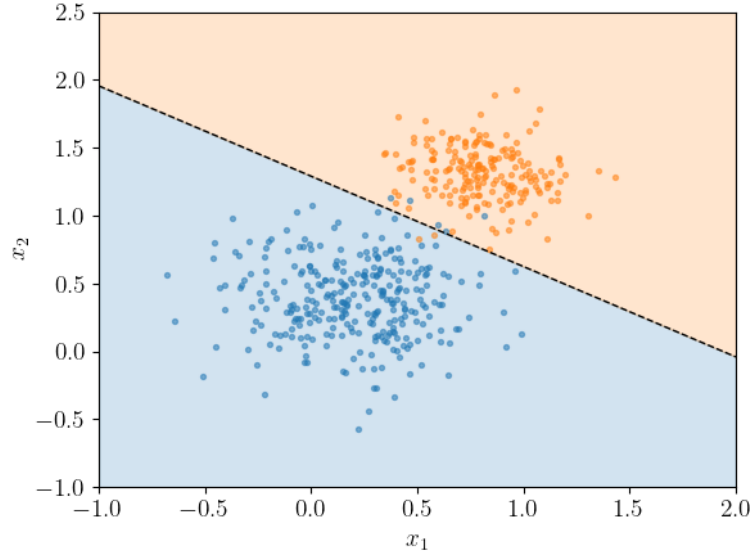
Hình 2.1: Hồi quy Logistic học một đường thẳng (hoặc siêu phẳng trong không gian nhiều chiều) để phân chia dữ liệu thành các lớp.
