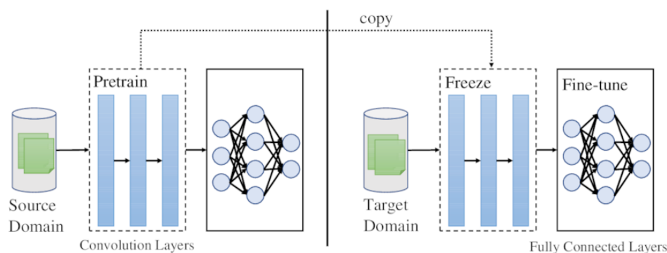
Hình 5.1: Mô hình Học Chuyển giao trong NLP: Một mô hình được huấn luyện trước trên dữ liệu lớn, sau đó được tinh chỉnh trên một tác vụ cụ thể.
