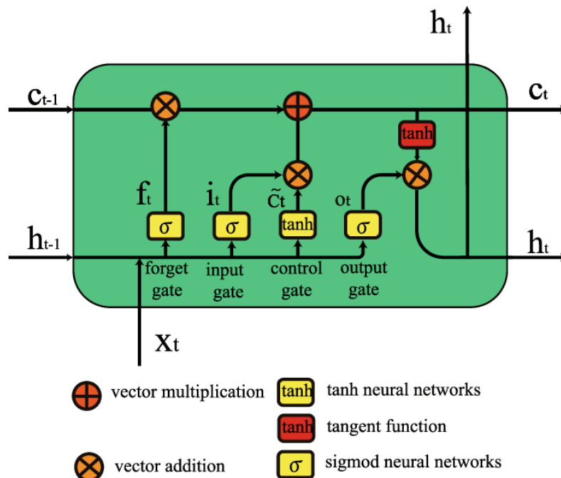
Hình 3.5: Sơ đồ chi tiết của một ô nhớ LSTM. Nó bao gồm 3 cổng chính (Quên, Nạp, Xuất) và một trạng thái ô nhớ C_t chạy ngang.
