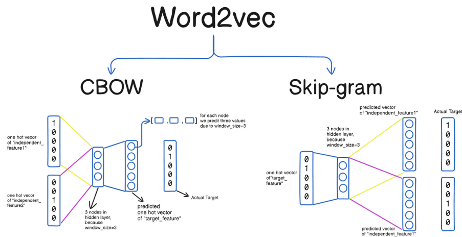
Hình 3.1: Kiến trúc chung của Word2Vec. Khi nhân vector one-hot của một từ với ma trận W , thực chất chúng ta đang "chọn" ra hàng tương ứng với từ đó, chính là vector embedding của nó. Ma trận W là mục tiêu chúng ta cần học.
