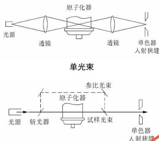
图 2 AAS 光路图
