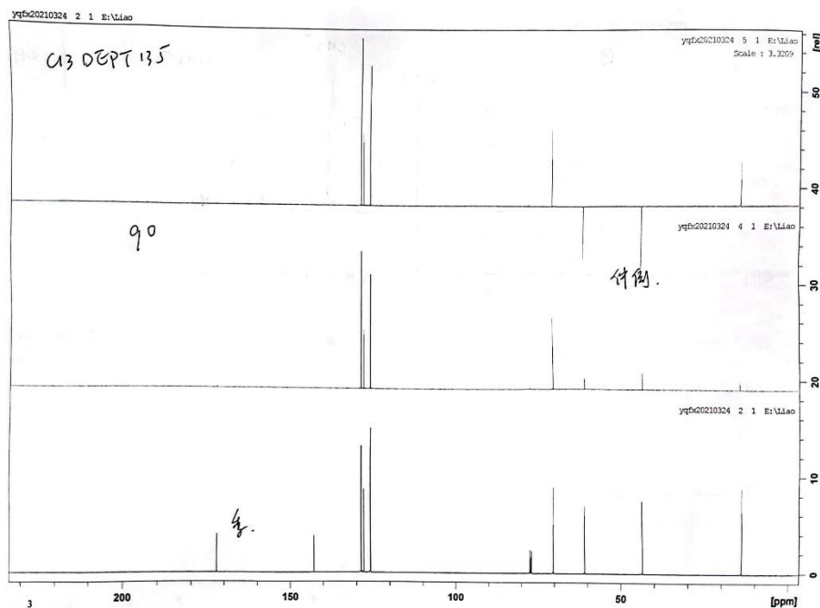
图 4 样品的 ^{13}\text{C}\{^1\text{H}\} -NMR 谱图、 ^{13}\text{C} DEPT90 谱图、 ^{13}\text{C} DEPT135 谱图对比
