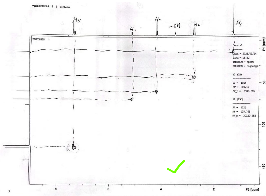
图 5 样品的 ^1\text{H} - ^{13}\text{C} HSQC 谱 (近程)
