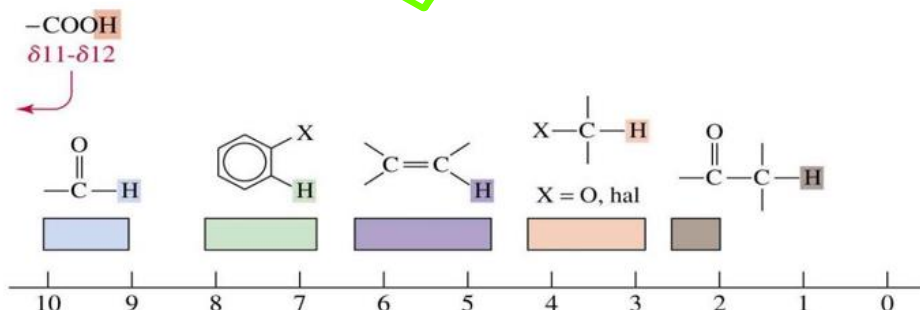
图 1 常见基团的 ^1\text{H} 化学位移值
