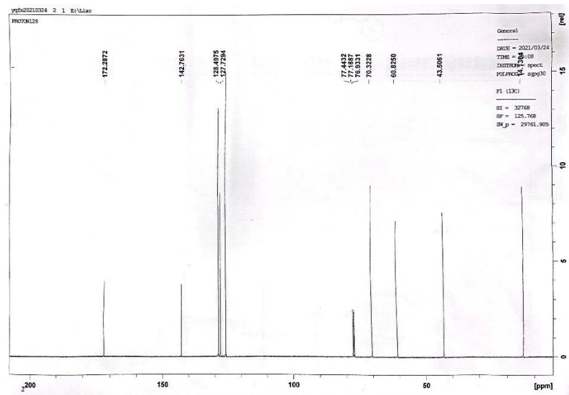
图 3 样品的 ^{13}\text{C}\{^1\text{H}\} -NMR 谱图
