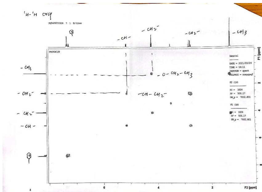
图 6 样品的 ^1\text{H} - ^1\text{H} COSY 谱图
