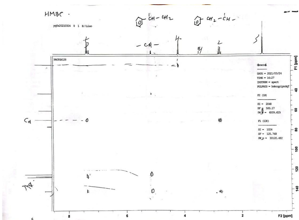
图 7 样品的 ^1\text{H} - ^{13}\text{C} HMBC 谱图
