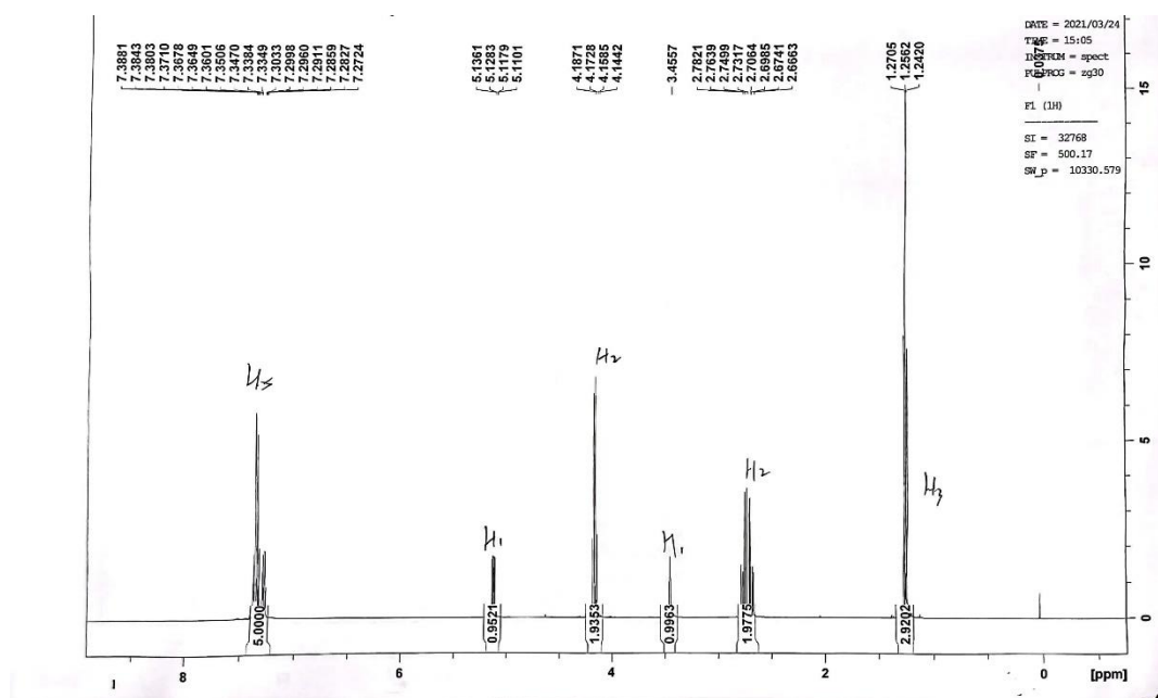
图 2 样品的 ^1H -NMR 谱图
