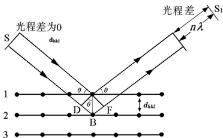
图 1 晶体产生 X 射线衍射的条件
