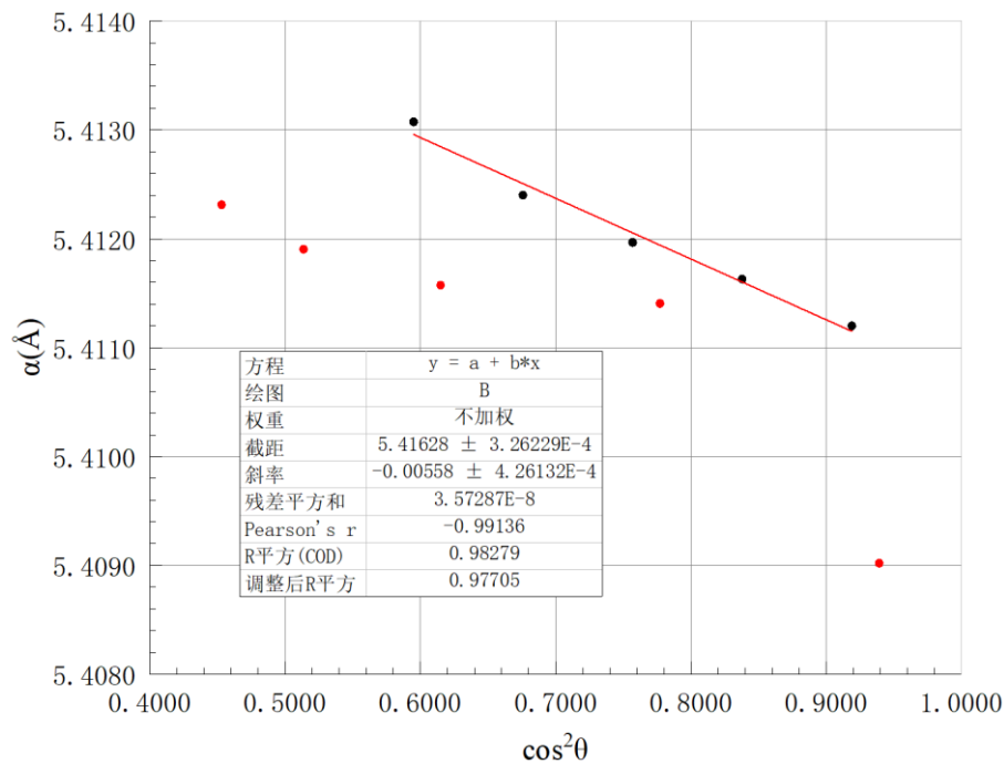
图 3 a \sim \cos^2\theta 拟合直线图
