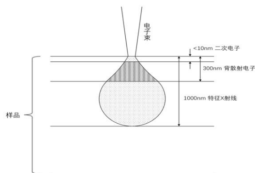
图 2 二次电子、背散射电子和特征 X 射线来源
