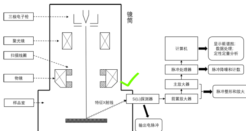
图 4 能谱仪的工作原理和基本结构
