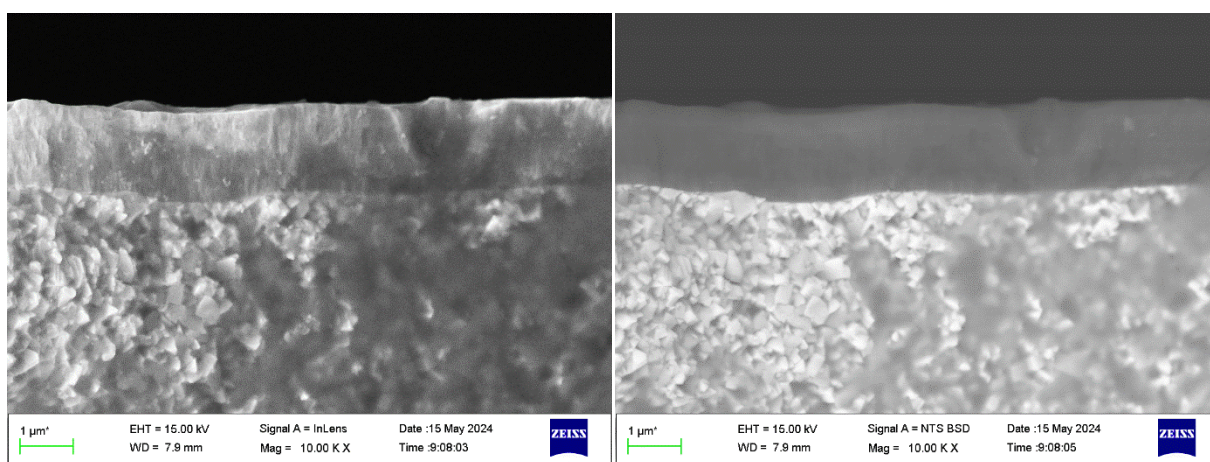
图 7 InLens 探头及 NTS BSD 探头下不锈钢钻头横截面电镜图
