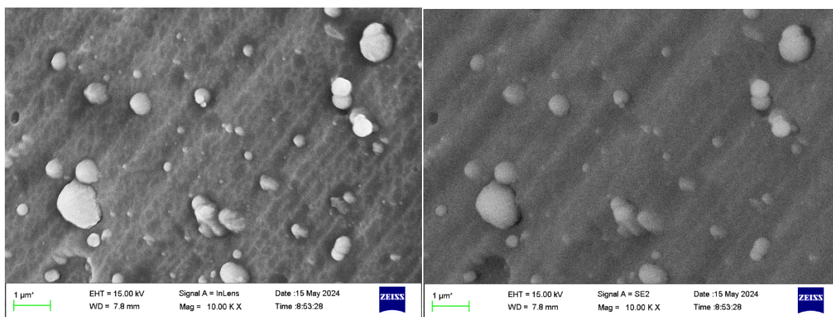
图 6 InLens 探头及 SE2 探头下不锈钢钻头表面电镜图
