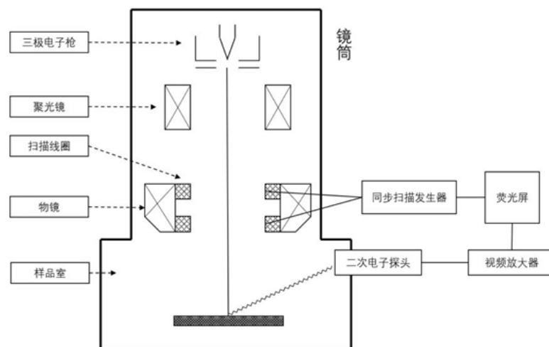
图 3 扫描电镜的基本结构
