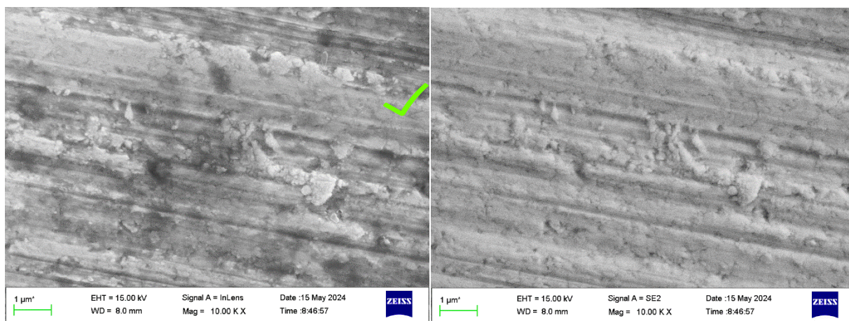
图 5 InLens 探头及 SE2 探头下不锈钢钻头表面电镜图
