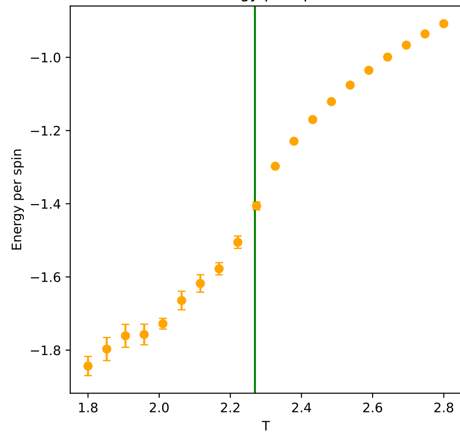
Energy per spin
