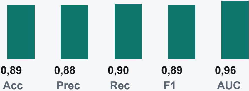
Regressão Logística
