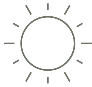
Éclaircie
