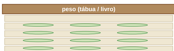
Figura 3. Secagem entre jornais com peso, recurso para envios demorados de material fúngico/morfológico (confirme com o laboratório).
