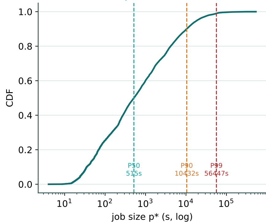
A. Job-size CDF
