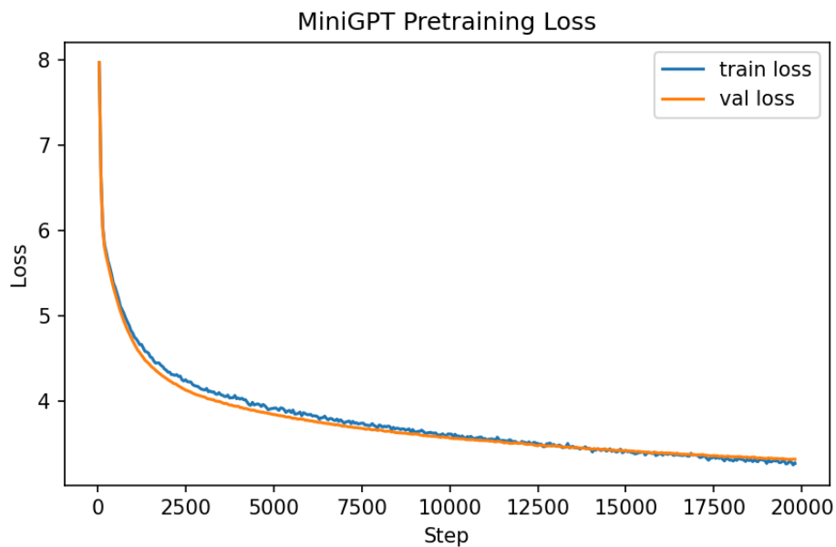
图 4-1 MiniGPT 在 TinyStories 数据集上的预训练 loss 曲线
