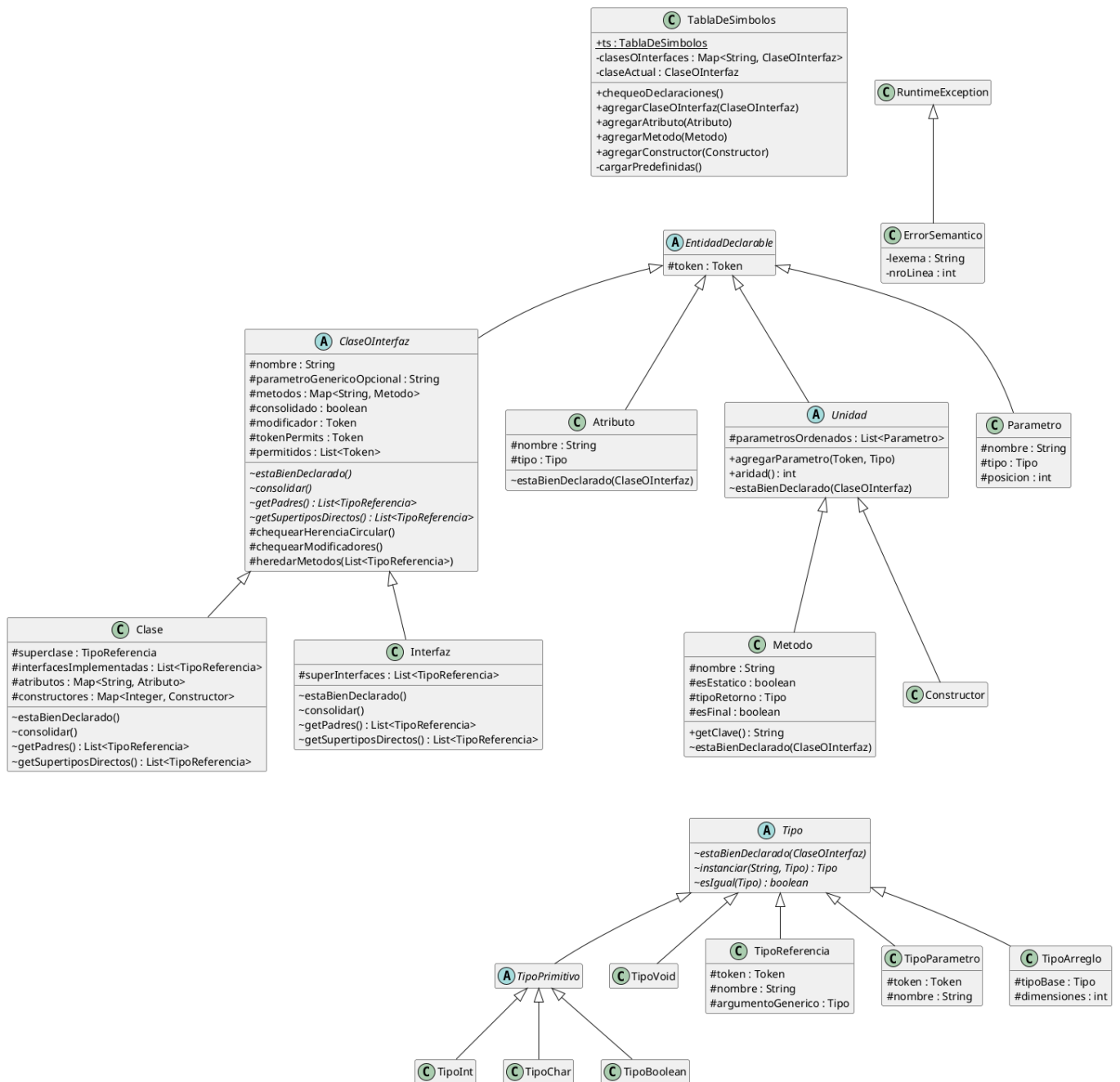
Diagrama de clases del analizador semántico
