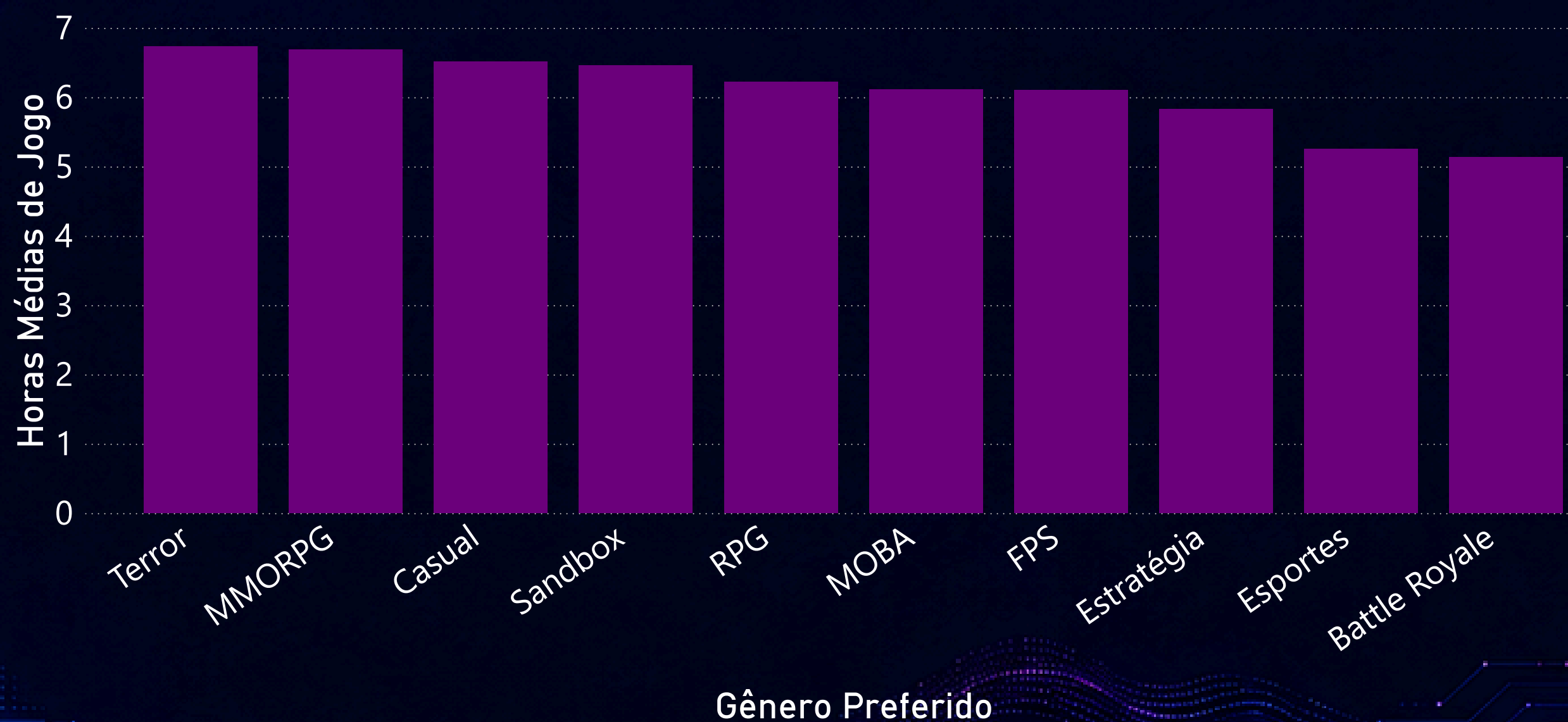
Horas Médias de Jogo por Gênero Preferido
