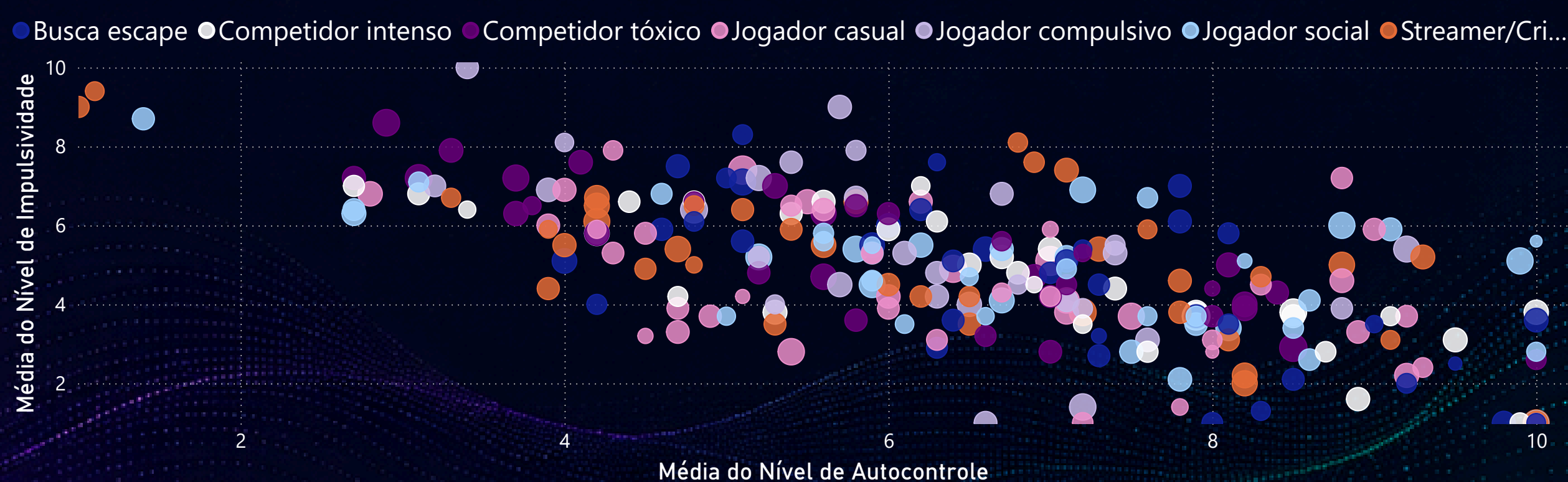
Autocontrole vs Impulsividade por Perfil Comportamental
