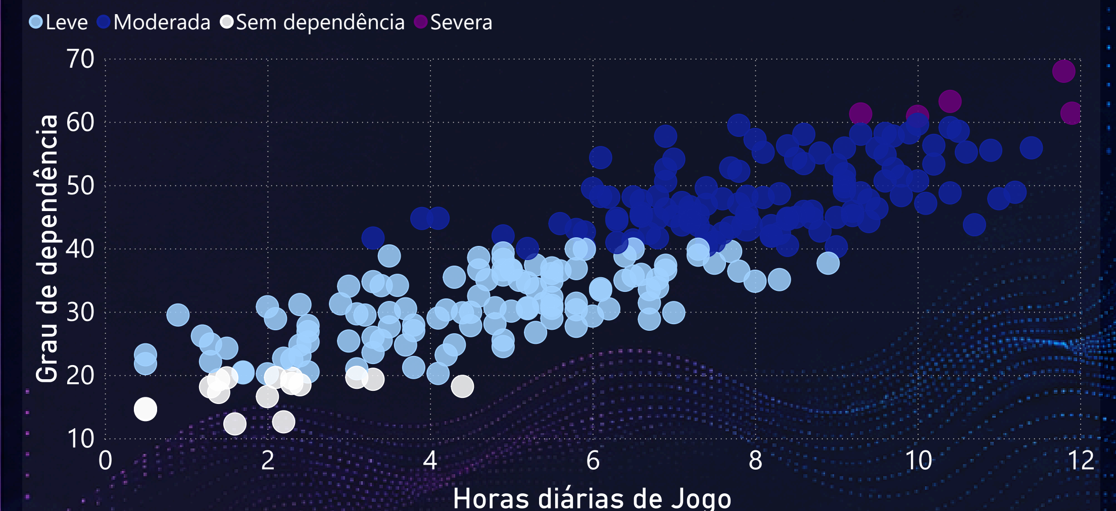
Horas de Jogo x Dependência e Risco à Saúde Mental
