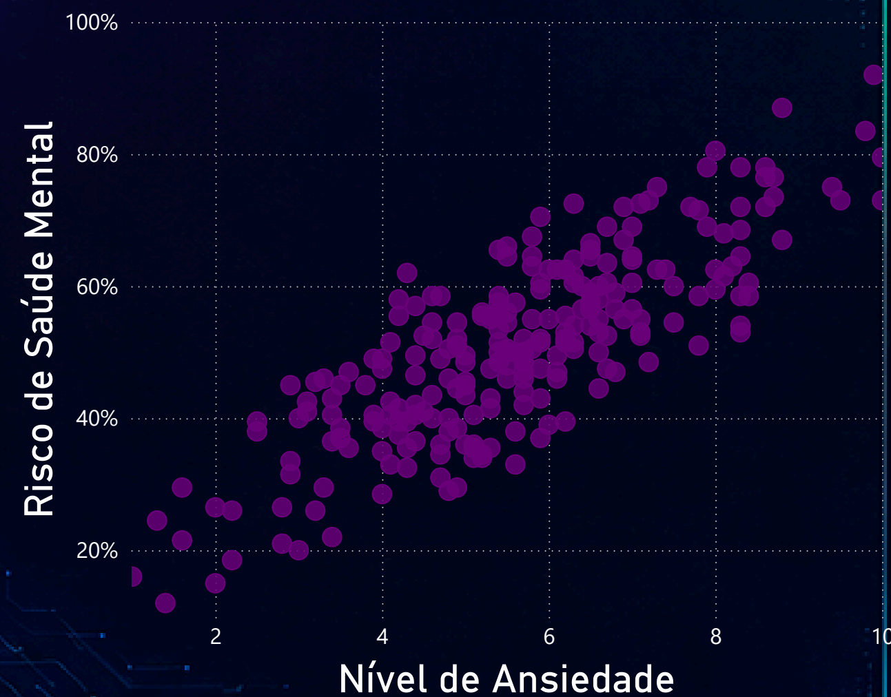
Nível de Ansiedade vs Risco de Saúde Mental
