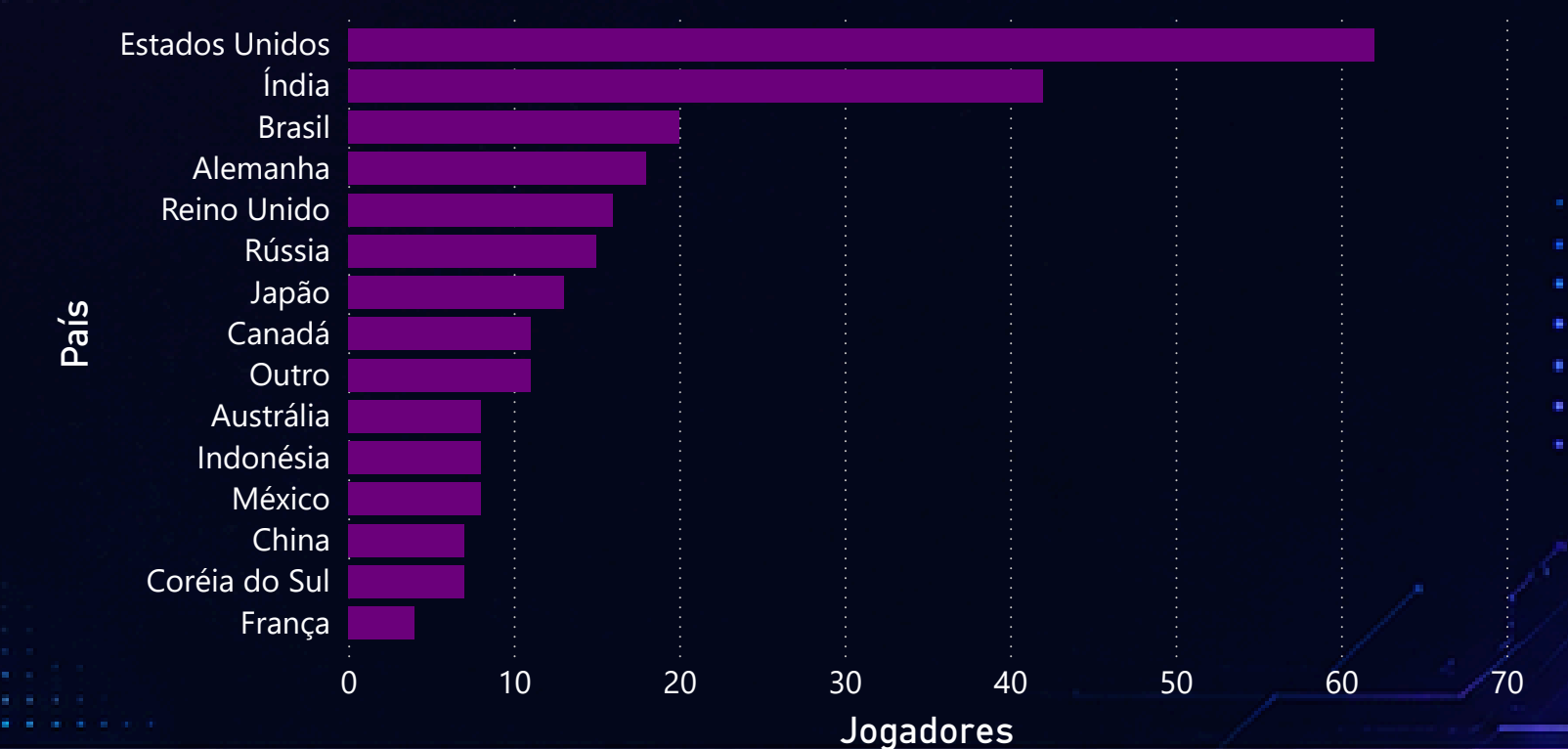
Jogadores por País
