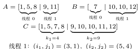
图 13.4: 协同秩函数的执行示例
