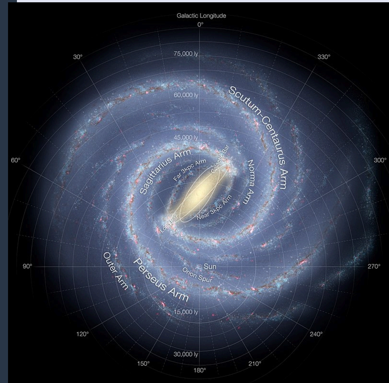
Ilustración de la Vía Láctea - 250 miles de millones de estrellas Crédito: NASA/JPL-Caltech/ESO/R. Hurt
