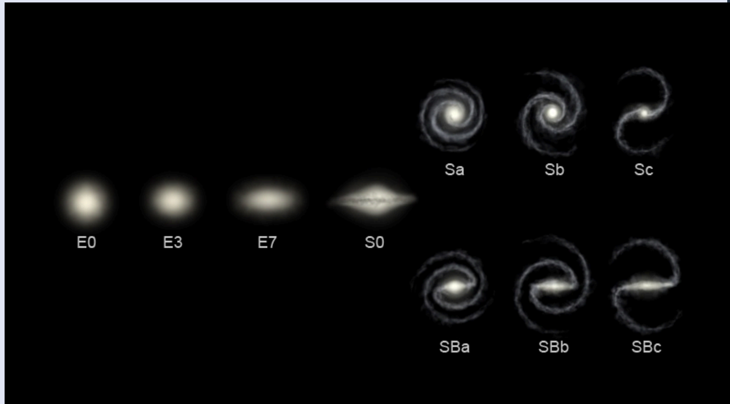
Diagrama en diapasón de la secuencia de Hubble. Créditos: Ikonact
