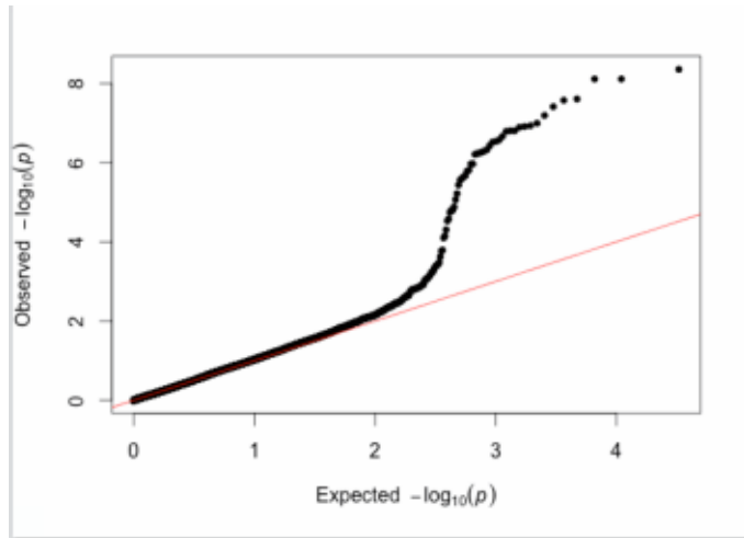
Q-Q
