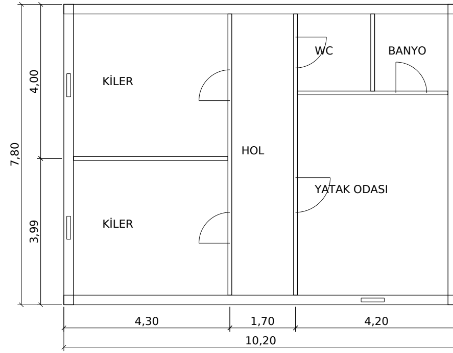
BODRUM KAT PLANI ÖLÇEK 1/100
