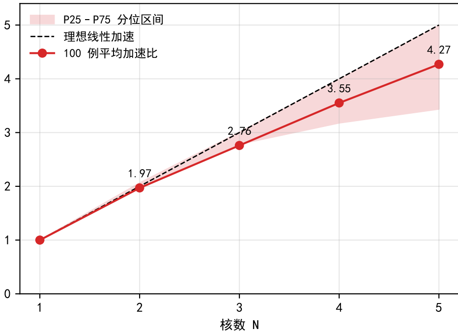
相对单核基准的平均加速比
