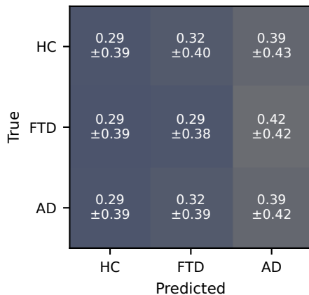
GPT-4o
