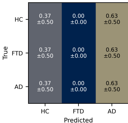
GPT-4.1-mini
