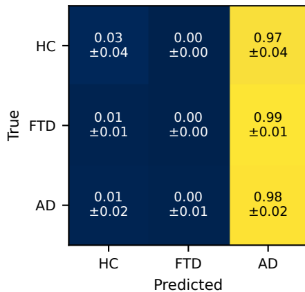
GLM-5
