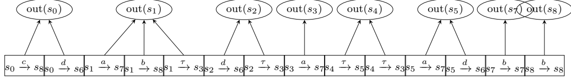
Fig. 5.15: La estructura (bySource), que representa la vista de transiciones ordenadas por estado de origen.
