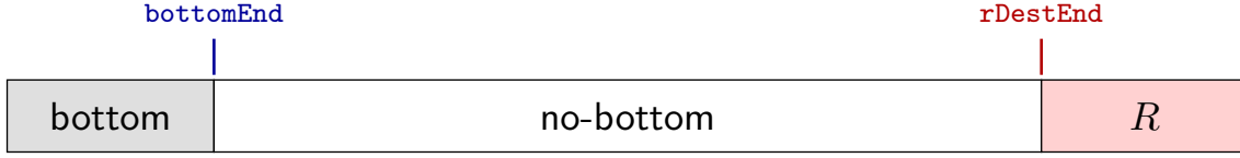
Fig. 5.6: Paso (c): addToR sobre un estado bottom .
