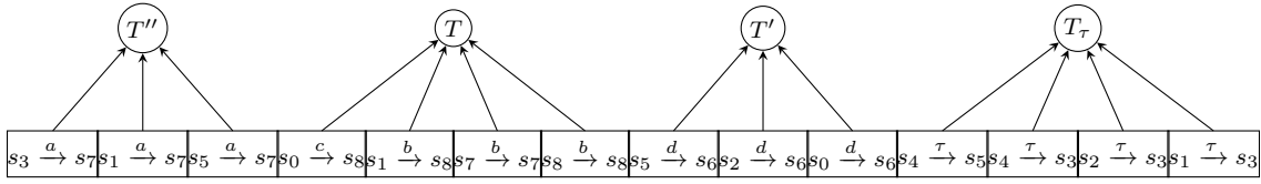
Fig. 5.13: La estructura de liveBunches, que representa la vista de todas las transiciones ordenadas por bunches de \Pi_t . Se usa el ejemplo de la Figura 5.1.
