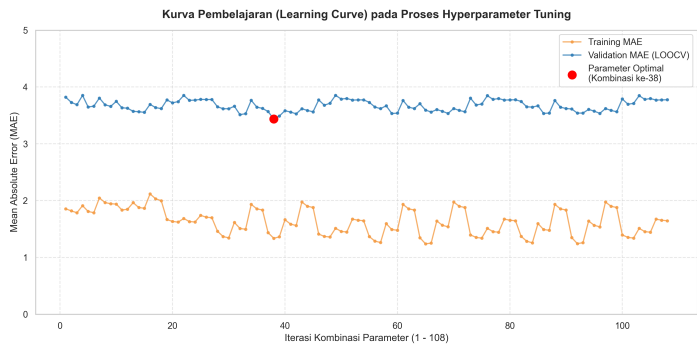
Gambar 5.4 Kurva Pelatihan dan Validasi pada Proses Hyperparameter Tuning
