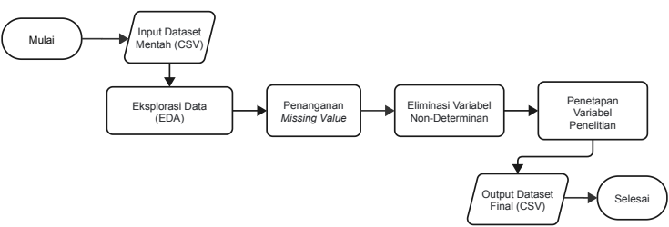
Gambar 3.3 Alur Pra-pemrosesan Data
