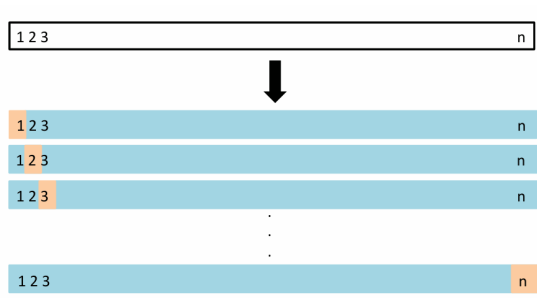
Gambar 2.3 Skema Partisi Data pada LOOCV james2023introduction
