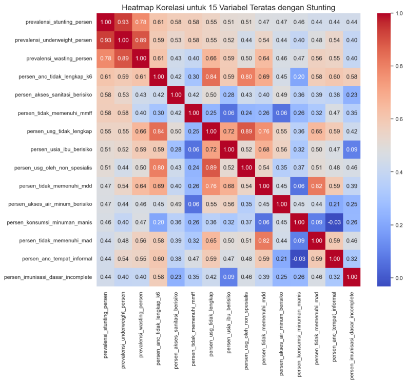
Gambar 5.3 Heatmap Korelasi 15 Variabel Teratas
