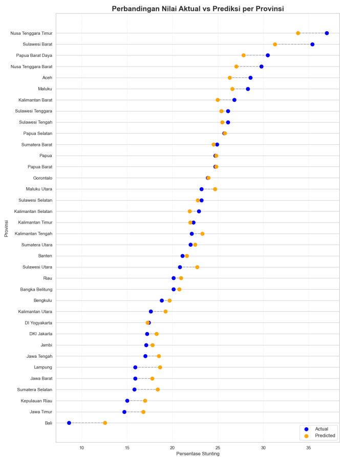
Gambar 5.5 Sebaran Nilai Aktual dan Prediksi Stunting per Provinsi
