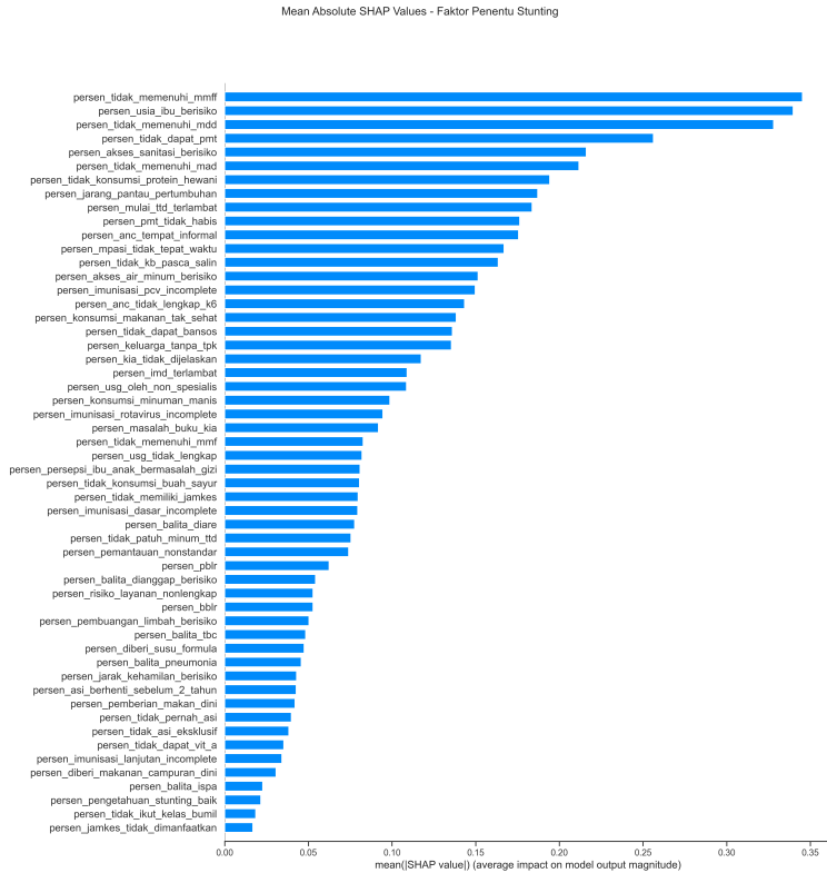
Gambar 3.1 Grafik Nilai Rata-Rata Absolut SHAP Seluruh Fitur
