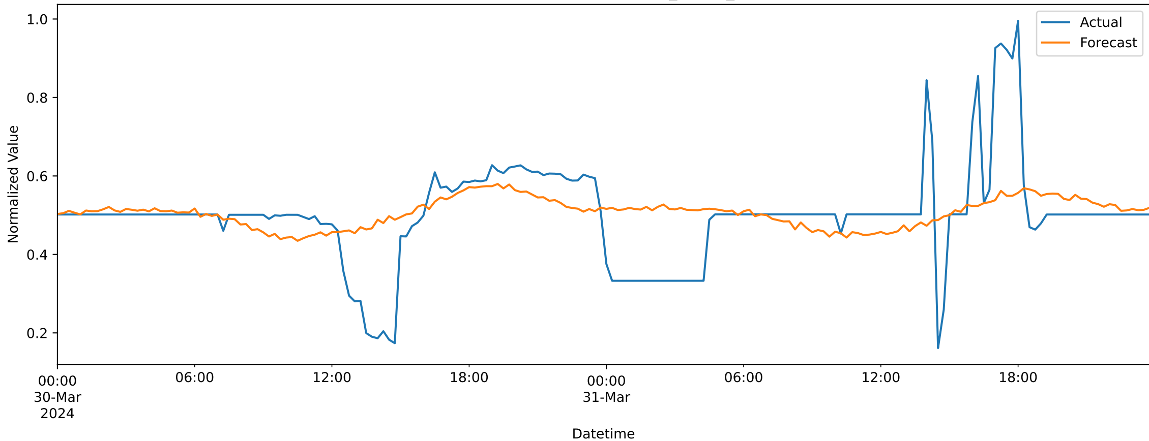
Forecast vs Actual - BESS_house_1
