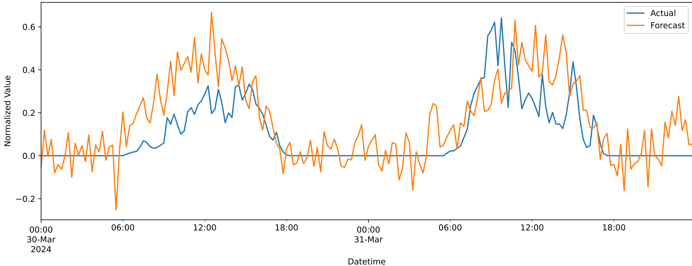
Forecast vs Actual - PV_house_4
