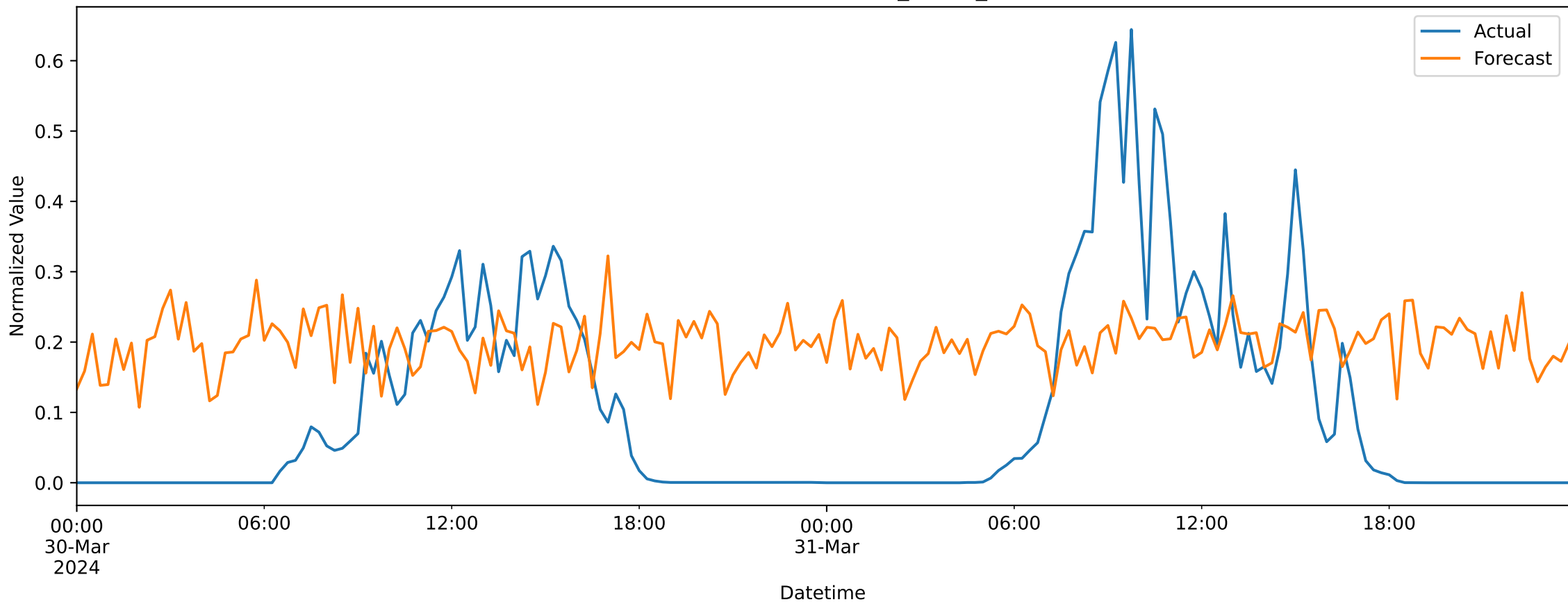
Forecast vs Actual - PV_house_1
