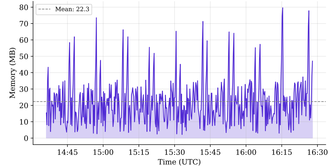
Heap — .NET
